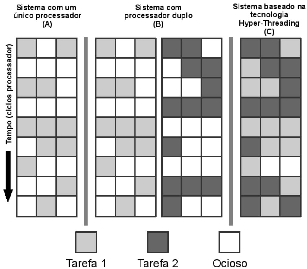
Figura 1.2: Comparativo de Execução dos Modelos Arquiteturais
