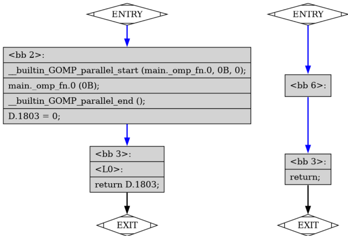
Figura 22.2: Representação Gráfica do Código GIMPLE
