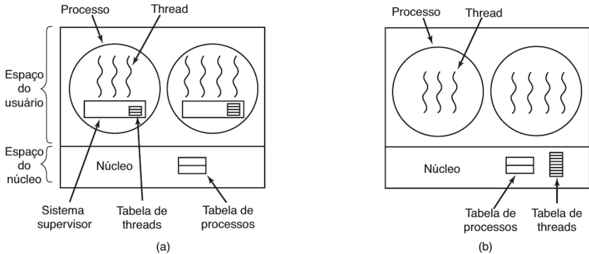
Figura 3.5: (a) Threads em nível de usuário. (b) Threads em nível de núcleo (Tanenbaum and Bos 2016).
