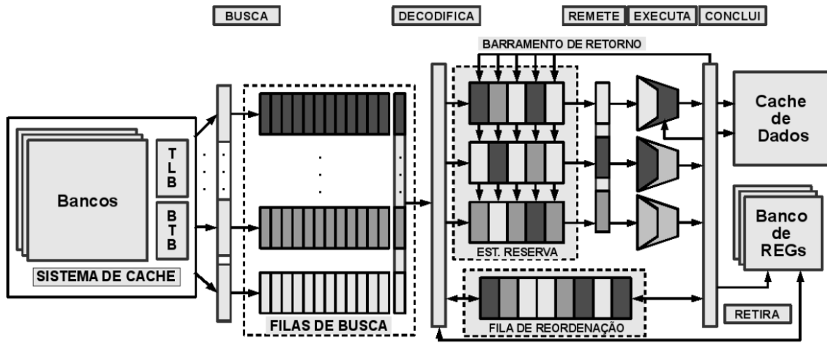
Figura 1.1: SMT
