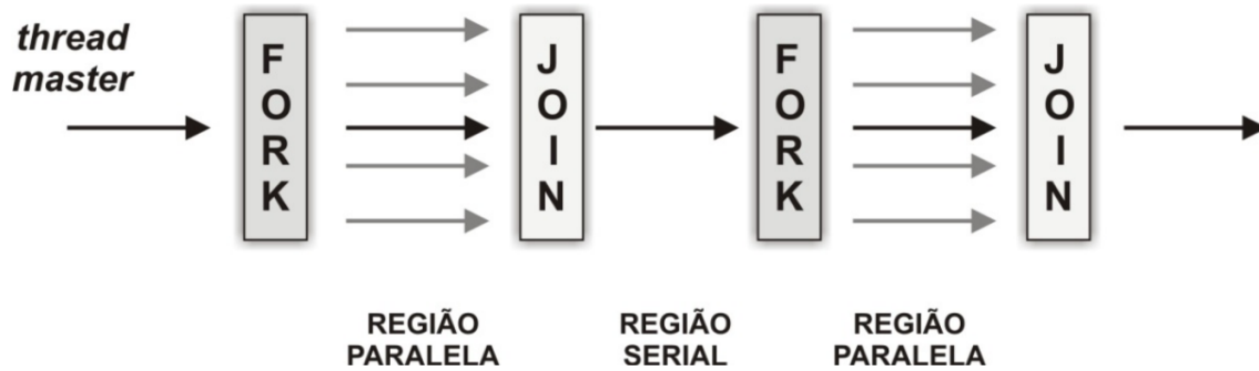
Figura 18.1: Modelo fork-join
