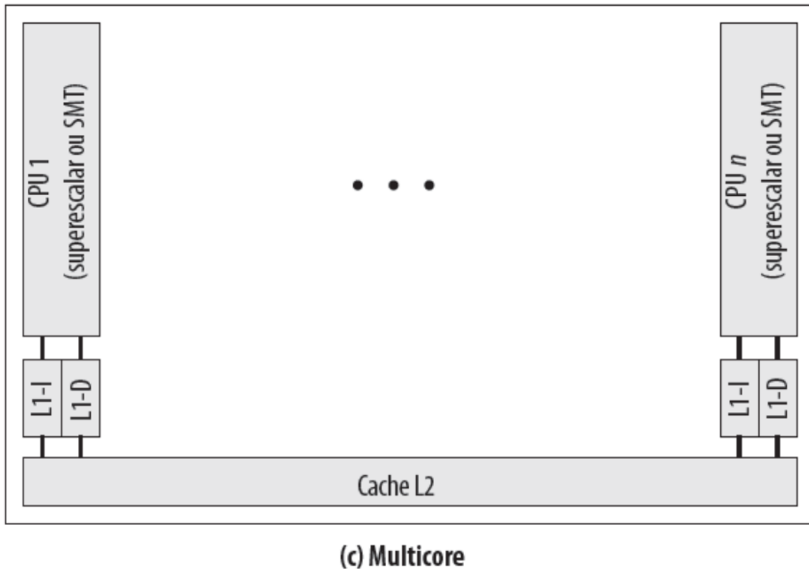
Figura 1.3: Multicore
