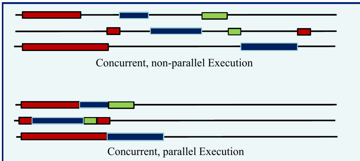
Figura 2.2: Concorrência e Paralelismo
