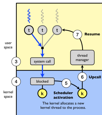
Figura 3.8: Ativação de escalonador via upcalls 2 .
