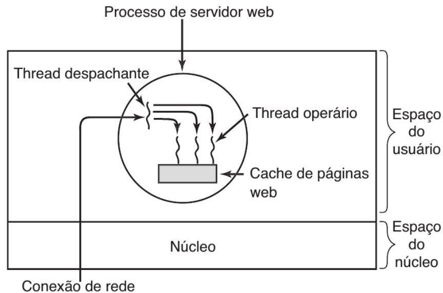
Figura 3.2: Servidor Web atendendo múltiplas requisições simultâneas (Tanenbaum and Bos 2016).
