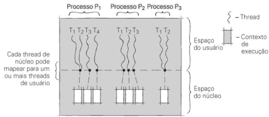
Figura 3.6: Mapeamento de Threads
