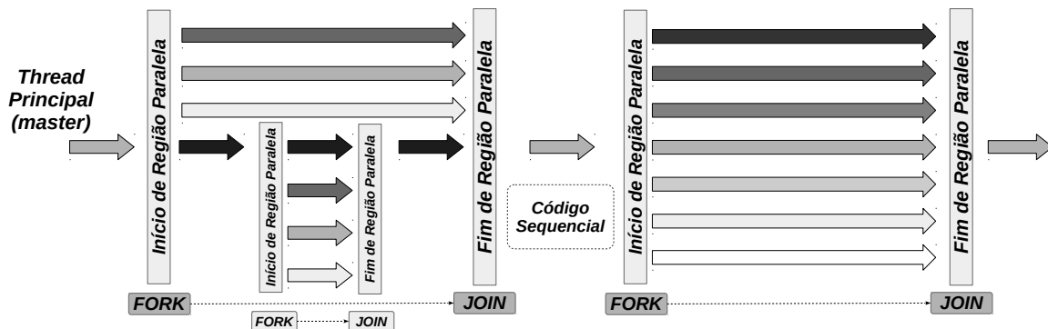
Figura 18.2: Modelo fork-join
