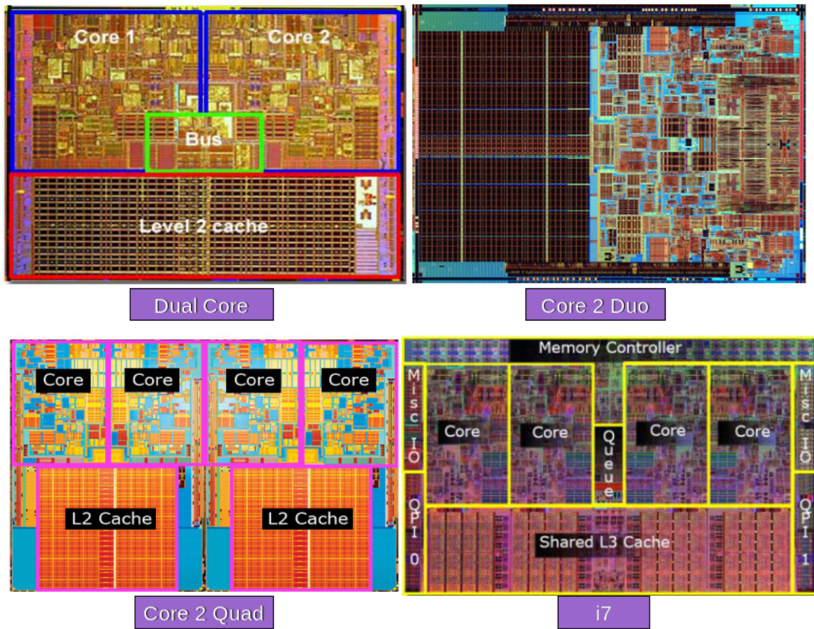
Figura 1.4: Multicore
