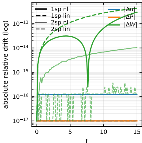
(d) 2 species (sp) vx-slices
