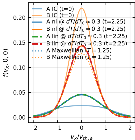
(d) 2 species (sp) vx-slices
