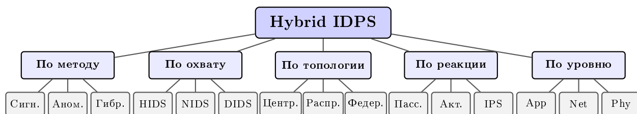
Рис. 1.1 – Иерархическая классификация Hybrid IDPS по пяти ортогональным осям. По методу обнаружения — сигнатурные (детерминированный поиск по базе известных шаблонов), аномалийные (статистическое или обучаемое отклонение от нормального профиля) и гибридные (комбинация обоих). По охвату — хостовые (HIDS), сетевые (NIDS) и распределённые (DIDS). По топологии развёртывания — централизованные, распределённые, федеративные. По характеру реагирования — пассивные (только оповещение), активные (вмешательство в поток), IPS (полная блокировка). По уровню стека — прикладной, сетевой и физический.
