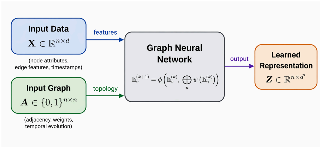
Рис. 1 – Двойственная природа входов моделей ГНС. Модель одновременно получает числовые данные (матрица признаков \mathbf{X} ) и реляционную структуру (матрица смежности \mathbf{A} ) в качестве входов. Возмущение любого из входов может нарушить обученное представление, что мотивирует разработку системы робастности, реализуемой в гибридных системах обнаружения и предотвращения вторжений, являющихся предметом настоящей диссертации.
