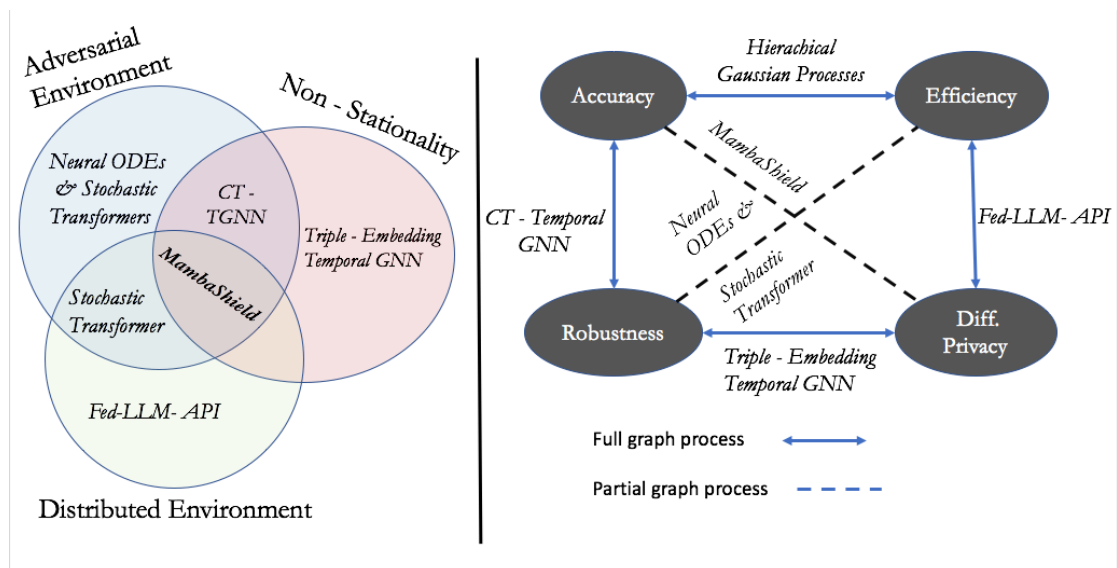
Рис. 2 – Расположение семи методов в пространстве условий функционирования (слева) и требований (справа). М4: MambaShield находится на пересечении всех трёх условий; М1: CT-TGNN связывает состязательное и нестационарное условия через сертифицированные непрерывно-временные динамики.
