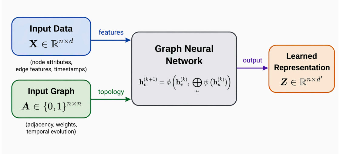
Рис. 1 – Двойственная природа входов ГНС-моделей, применяемых в качестве одной из ветвей обучаемых детекторов в системах Hybrid IDPS. Модель одновременно получает числовые данные (матрица признаков \mathbf{X} ) и реляционную структуру (матрица смежности \mathbf{A} ). Возмущение любого из входов может нарушить обученное представление, что мотивирует разработку системы повышения робастности и эффективности Hybrid IDPS, являющейся предметом настоящей диссертации.
