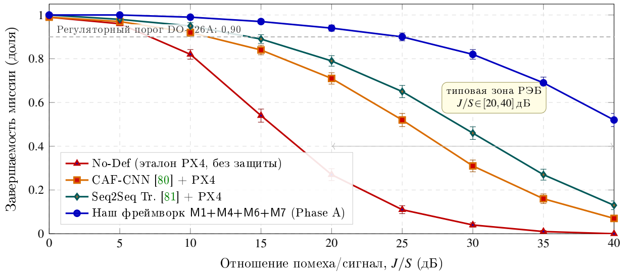
Рис. 6.7 – Завершаемость миссии БПЛА в зависимости от интенсивности РЭБ-подавления, измеренной как отношение мощности помехи к мощности полезного сигнала ( J/S , дБ). Эталон UAV-EW-Bench-2026: 5 000 симулированных вылетов (AirSim / PX4 SITL), три типа миссий, три модели ГНСС-приёмника, комбинированный состязательный контур. Полосы ошибок — 95 % доверительные интервалы Уилсона ( n = 200 на точку, три зёрна). Предлагаемый фреймворк М1+М4+М6+М7 удерживает завершаемость выше регуляторного порога DO-326A 0,90 до J/S \approx 27 дБ включительно — против \approx 18 дБ для Seq2Seq Tr., \approx 13 дБ для CAF-CNN и \approx 7,5 дБ для эталонной PX4 без защиты, то есть выигрыш в 9–19 дБ по операционно-значимому показателю.
