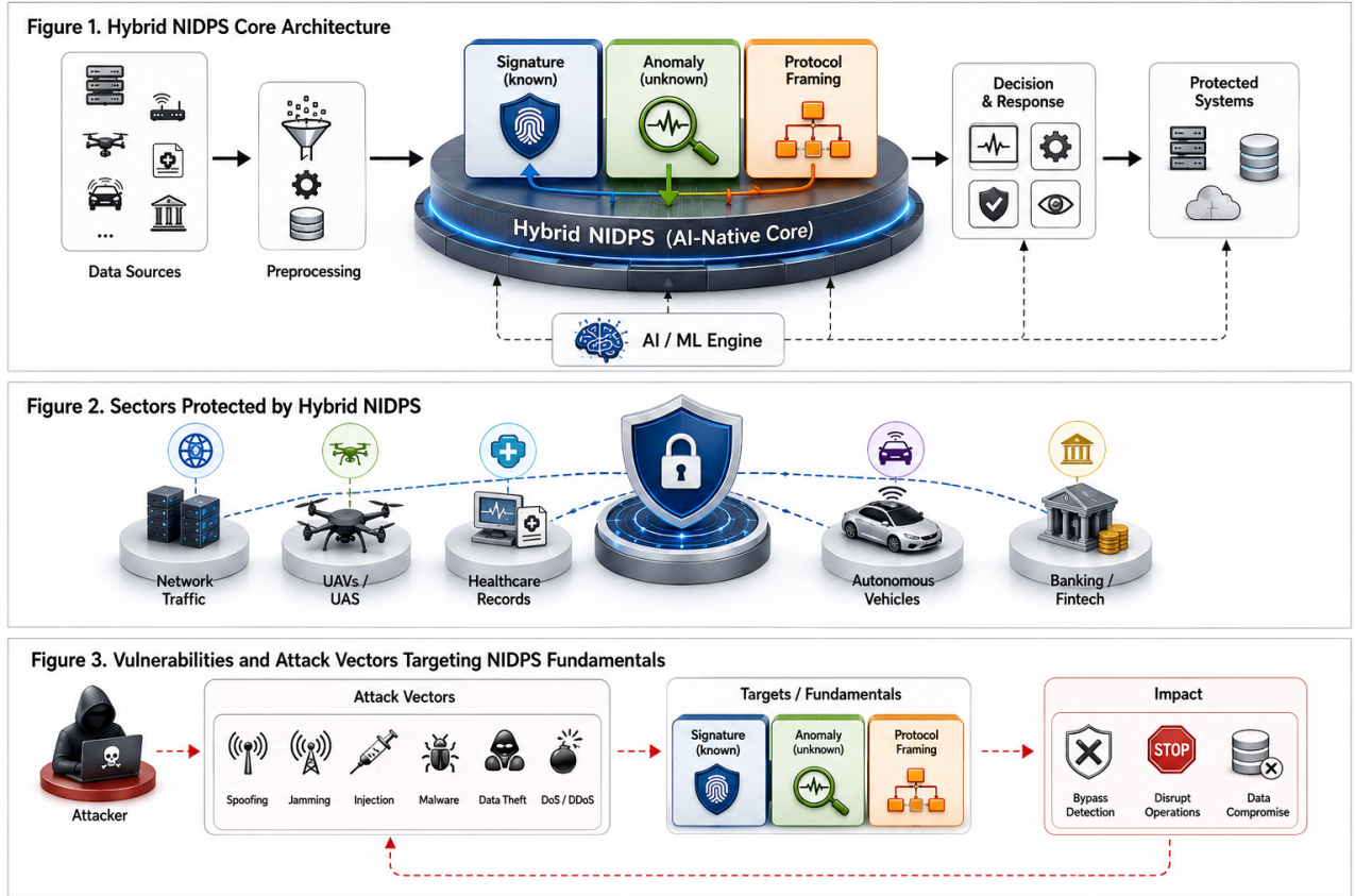
Рис. 1 – Концептуальная схема гибридной СОПВ в трёх аспектах. Сверху — ядро архитектуры (Hybrid NIDPS AI-Native Core) с трёхканальным детектированием (сигнатурный, аномалийный, протокольный), AI/ML-движком в качестве усиливающего слоя, блоком принятия решений и реагирования и защищаемыми системами. В центре — предметные области применения системы: сетевой трафик, БПЛА, медицинские записи, автономные транспортные средства, банковско-финансовая инфраструктура. Снизу — поверхность атак на канонические компоненты: атакующий → векторы атак (спуфинг, джемминг, инъекция, malware, утечка данных, DoS/DDoS) → целевые компоненты (signature, anomaly, protocol framing) → последствия (обход обнаружения, нарушение работы, компрометация данных).
