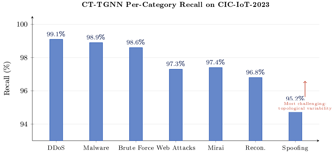
Рис. 4.2 – Покатегорийная полнота CT-TGNN на CIC-IoT-2023 по семи основным семействам атак. DDoS достигает наивысшей полноты (99,1%), тогда как спуфинг наиболее сложен (95,2%), что отражает его большую топологическую вариативность.
