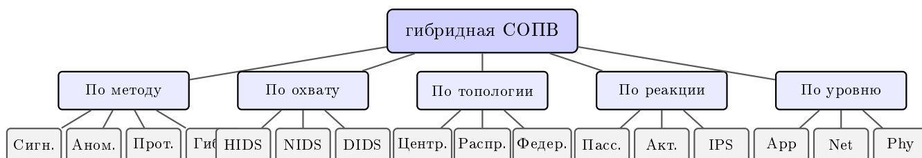
Рис. 1.2 – Иерархическая классификация гибридная СОПВ по пяти ортогональным осям. По методу обнаружения — сигнатурные (детерминированный поиск по базе известных шаблонов), аномалийные (статистическое или обучаемое отклонение от нормального профиля), протокольные (контекстно-зависимый анализ корректности сетевых, прикладных и промышленных протоколов и их состояний) и гибридные (комбинация трёх предыдущих, усиленная обучаемыми моделями M1–M7). По охвату — хостовые (HIDS), сетевые (NIDS) и распределённые (DIDS). По топологии развёртывания — централизованные, распределённые, федеративные. По характеру реагирования — пассивные (только оповещение), активные (вмешательство в поток), IPS (полная блокировка). По уровню стека — прикладной, сетевой и физический.
