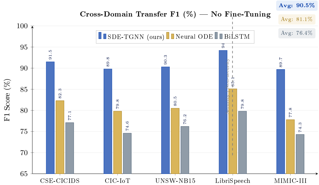
Рис. 4.7 – Кросс-доменный перенос F1 (%) для SDE-TGNN, базовой линии Neural ODE и базовой линии BiLSTM на трёх наборах данных безопасности и двух областях вне безопасности (речь, здравоохранение). SDE-TGNN достигает 90,5% среднего переноса без дообучения, что на 9,4 п. п. выше Neural ODE и на 14,1 п. п. выше BiLSTM.
