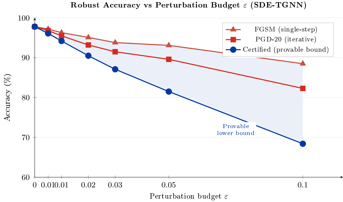
Рис. 4.6 – Робастная точность как функция бюджета возмущений \epsilon для FGSM, PGD-20 и сертифицированных (рандомизированное сглаживание) оценок SDE-TGNN. Сертифицированная кривая обеспечивает доказуемую нижнюю границу; FGSM и PGD представляют эмпирические верхние границы при конкретных стратегиях атак.
