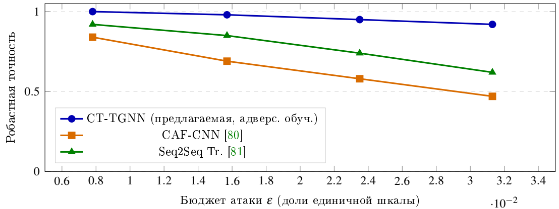
Рис. 6.5 – Зависимость робастной точности от бюджета PGD-атаки \varepsilon для трёх архитектур. Предлагаемая СТ-TGNN сохраняет робастную точность \geq 0,92 во всём исследуемом диапазоне.
