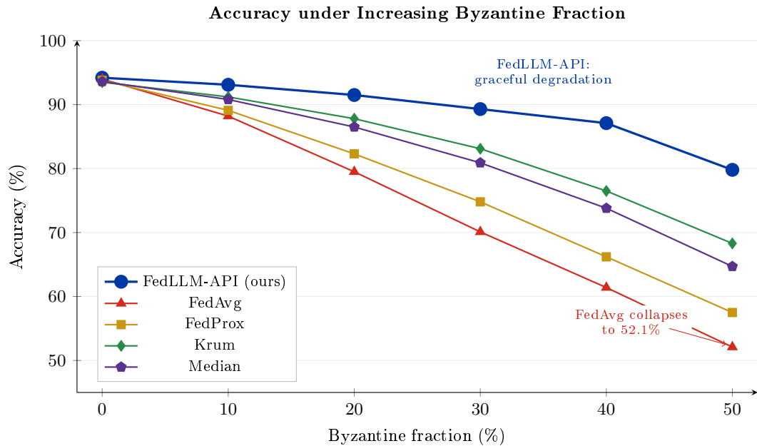
Рис. 4.4 – Дegradaция точности FedLLM-API при увеличении доли византийских участников в сравнении с базовыми линиями FedAvg, FedProx, Krum и Медиана. FedLLM-API плавно деградирует с 94,2% до 79,8% при увеличении повреждения с 0% до 50%, тогда как FedAvg обрушивается до 52,1%.
