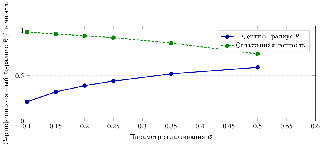
Рис. 6.6 – Компромисс между параметром сглаживания \sigma , сертифицированным \ell_2 -радиусом и точностью сглаженного классификатора (Cohen-style, \alpha = 10^{-3} ).
