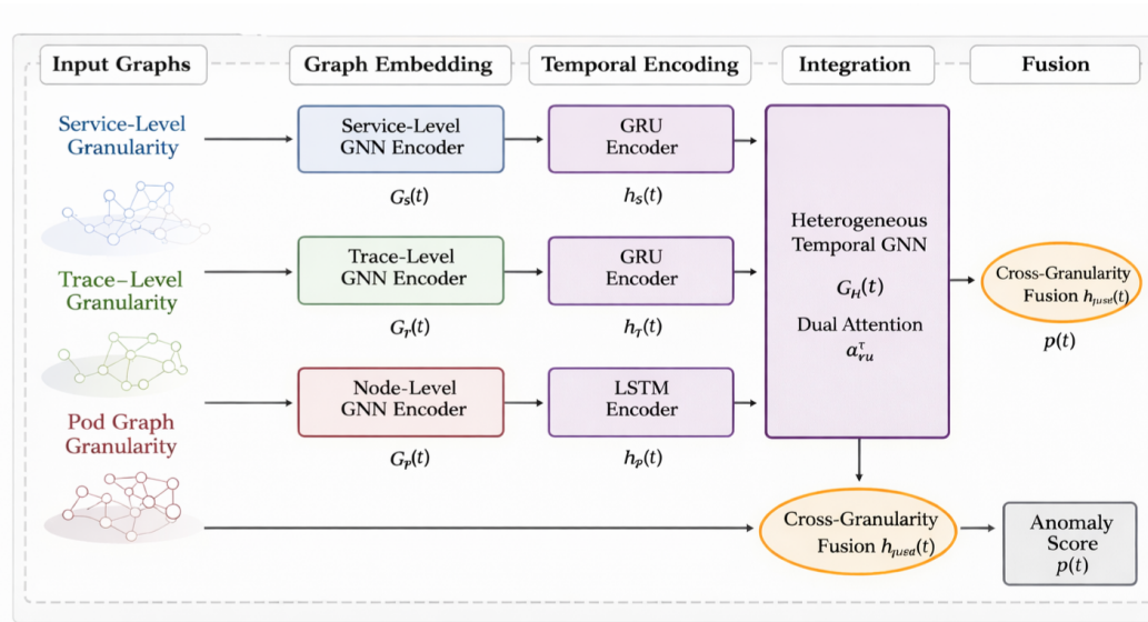
Рис. 3.3 – Архитектура TripleE-TGNN для многоуровневого мониторинга безопасности в облачных средах.
