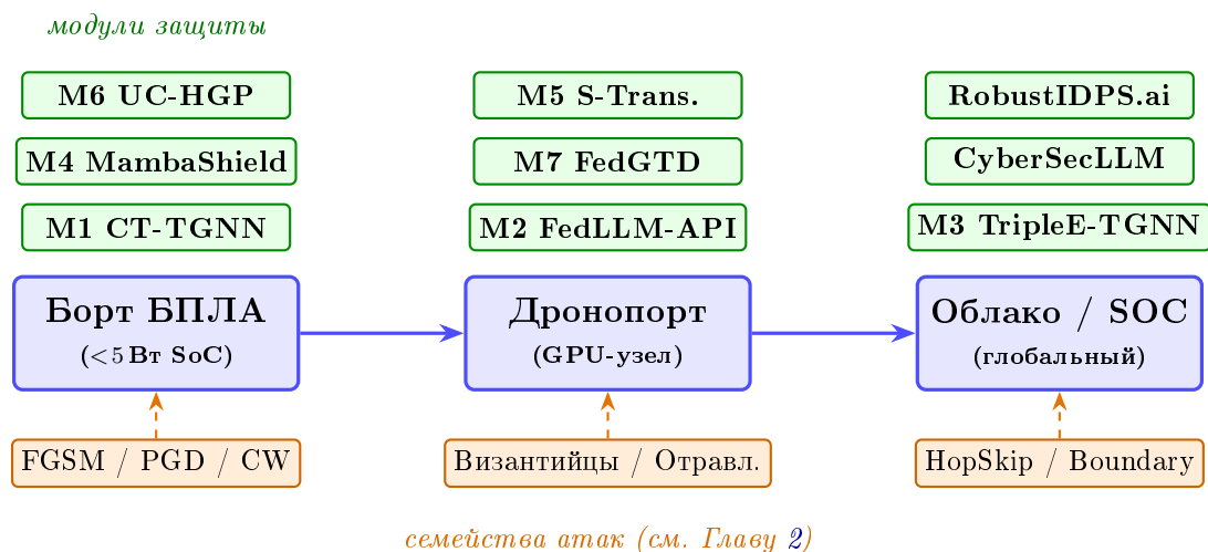
Рис. 6.3 – Трёхуровневая архитектура единого защитного фреймворка для нейросетевой системы навигации БПЛА. Методы M1–M7 и фундаментальная модель CyberSecLLM распределены по уровням борт — дронпорт — облако в соответствии с их вычислительной сложностью и сетевыми ограничениями.
