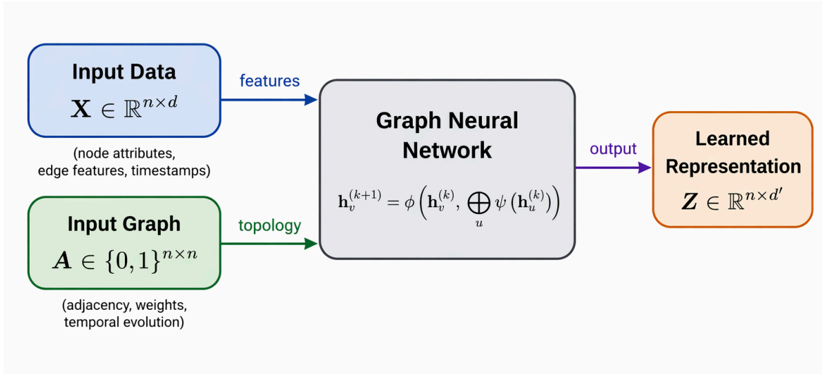
Рис. 2 – Двойственная природа входов ГНС-моделей, применяемых в качестве одной из ветвей обучаемых детекторов в системах гибридных СОПВ. Модель одновременно получает числовые данные (матрица признаков \mathbf{X} ) и реляционную структуру (матрица смежности \mathbf{A} ). Возмущение любого из входов может нарушить обученное представление, что мотивирует разработку системы повышения робастности и эффективности гибридных СОПВ, являющейся предметом настоящей диссертации.
