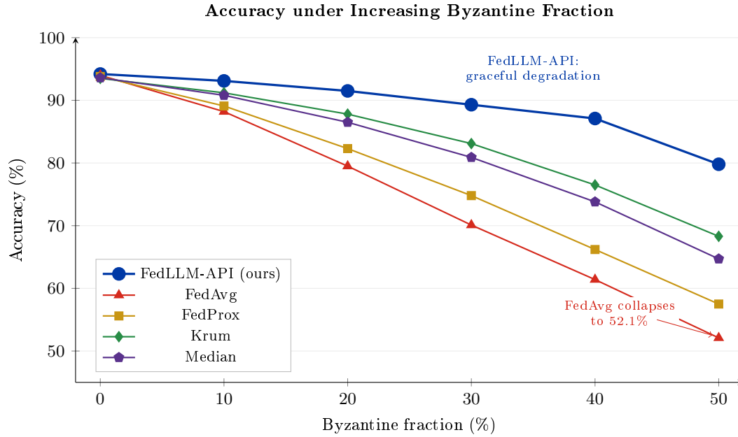
Рис. 4.4 – Дegradaция точности FedLLM-API при увеличении доли византийских участников в сравнении с базовыми линиями FedAvg, FedProx, Krum и Медиана. FedLLM-API плавно деградирует с 94,2% до 79,8% при увеличении повреждения с 0% до 50%, тогда как FedAvg обрушивается до 52,1%.
