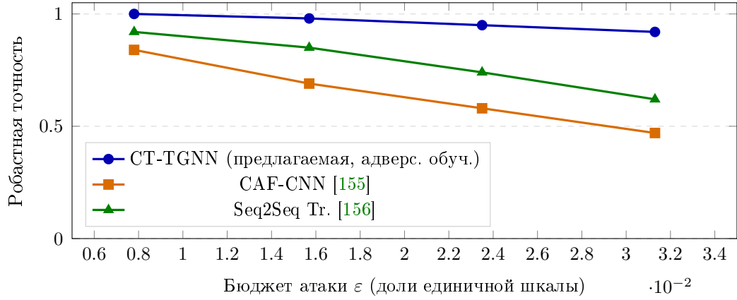
Рис. 6.5 – Зависимость робастной точности от бюджета PGD-атаки \epsilon для трёх архитектур. Предлагаемая СТ-TGNN сохраняет робастную точность \geq 0,92 во всём исследуемом диапазоне.
