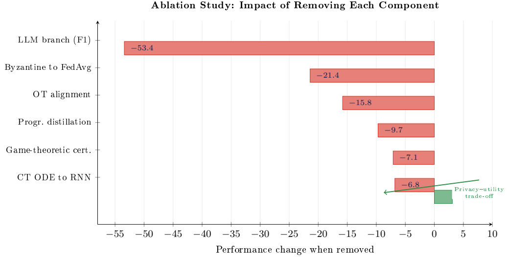
Рис. 4.5 – Абляционное исследование: падение производительности при удалении каждого компонента. Горизонтальные полосы показывают величину деградации; ветвь LLM, византийское усечённое среднее и выравнивание ОТ — три наиболее критичных компонента. Шум ДП — единственный компонент, удаление которого повышает точность (+3,1%), отражая компромисс приватность–качество.
