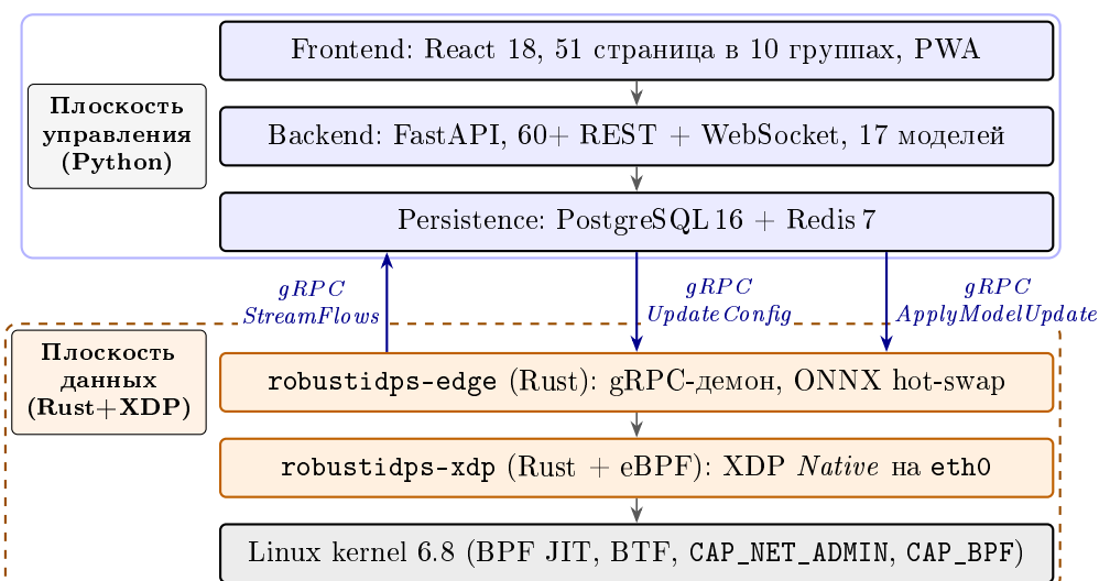
Рис. 5.3 – Двухплатформенная архитектура RobustIDPS.ai v4: Python-платформа управления (синяя рамка, верх) и Rust-платформа данных (оранжевая пунктирная рамка, низ) разделены чёткой границей и связаны тремя gRPC-примитивами. StreamFlows — поток записей о потоках из платформы данных в платформу управления; UpdateConfig — проталкивание списков блокировки в обратном направлении; ApplyModelUpdate — атомарная доставка INT8 ONNX-ученика на работающие агенты без перезапуска.
