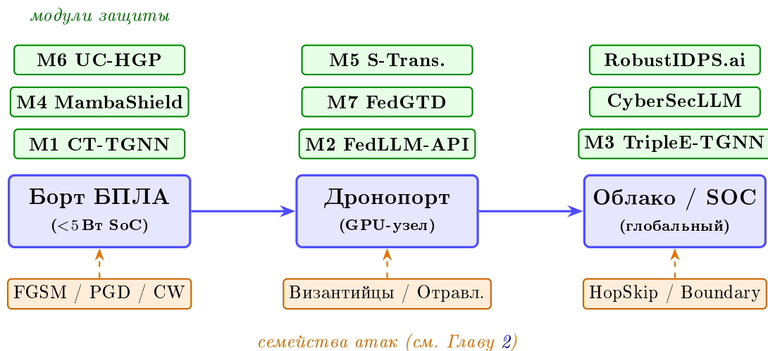
Рис. 6.3 – Трёхуровневая архитектура единого защитного фреймворка для нейросетевой системы навигации БПЛА. Методы M1–M7 и фундаментальная модель CyberSecLLM распределены по уровням борт — дронепорт — облако в соответствии с их вычислительной сложностью и сетевыми ограничениями.
