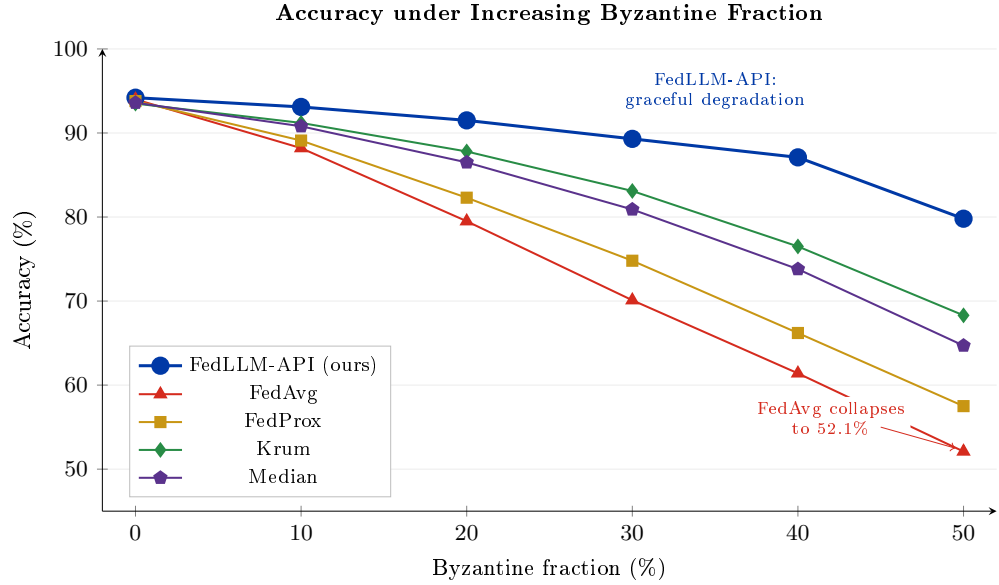
Рис. 4.4 – Деградация точности FedLLM-API при увеличении доли византийских участников в сравнении с базовыми линиями FedAvg, FedProx, Krum и Медиана. FedLLM-API плавно деградирует с 94,2% до 79,8% при увеличении повреждения с 0% до 50%, тогда как FedAvg обрушивается до 52,1%.
