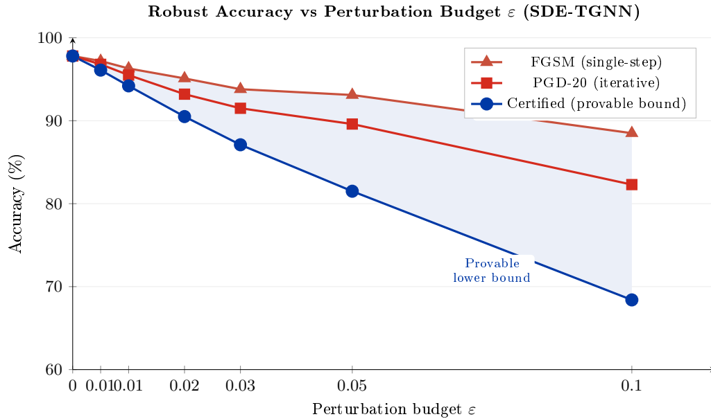
Рис. 4.6 – Робастная точность как функция бюджета возмущений \varepsilon для FGSM, PGD-20 и сертифицированных (рандомизированное сглаживание) оценок SDE-TGNN. Сертифицированная кривая обеспечивает доказуемую нижнюю границу; FGSM и PGD представляют эмпирические верхние границы при конкретных стратегиях атак.
