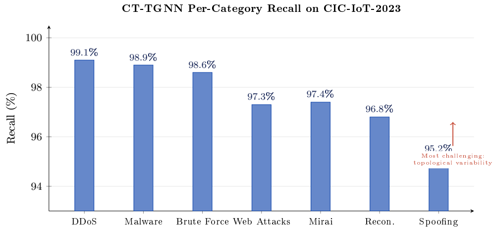
Рис. 4.2 – Покатегорийная полнота СТ-TGNN на CIC-IoT-2023 по семи основным семействам атак. DDoS достигает наивысшей полноты (99,1%), тогда как спуфинг наиболее сложен (95,2%), что отражает его большую топологическую вариативность.
