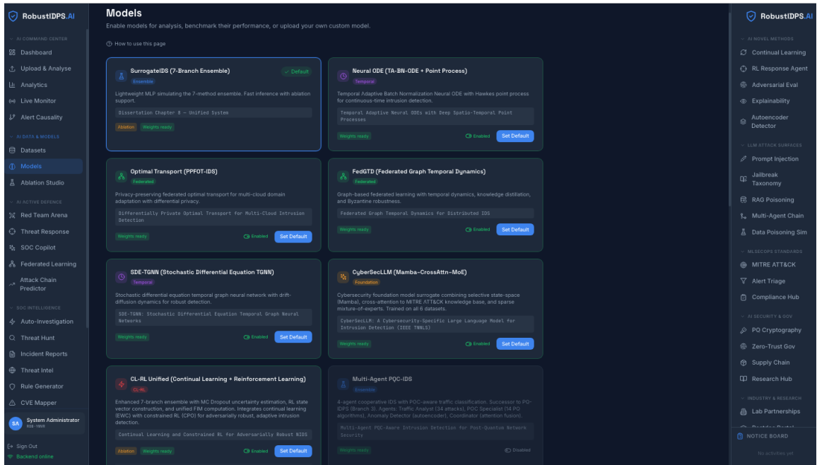
Рис. 5.4 – Страница моделей, отображающая 13+ интегрированных моделей обнаружения с настраиваемыми гиперпараметрами, метриками точности по каждой модели и бенчмарками задержки. Пользователи могут выбрать любую модель в качестве активного детектора или запустить ансамблевые сравнения.
