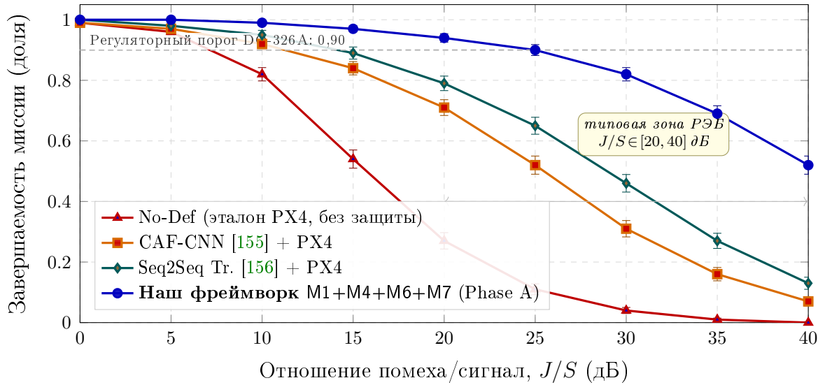
Рис. 6.4 – Завершаемость миссии БПЛА в зависимости от интенсивности РЭБ-подавления, измеренной как отношение мощности помехи к мощности полезного сигнала ( J/S , дБ). Эталон UAV-EW-Bench-2026: 5 000 симулированных вылетов (AirSim / PX4 SITL), три типа миссий, три модели ГНСС-приёмника, комбинированный состязательный контур. Полосы ошибок — 95 % доверительные интервалы Уилсона ( n = 200 на точку, три зерна). Предлагаемый фреймворк M1+M4+M6+M7 удерживает завершаемость выше регуляторного порога DO-326A 0,90 до J/S \approx 27 дБ включительно — против \approx 18 дБ для Seq2Seq Tr., \approx 13 дБ для CAF-CNN и \approx 7,5 дБ для эталонной PX4 без защиты, то есть выигрыш в 9–19 дБ по операционно-значимому показателю.
