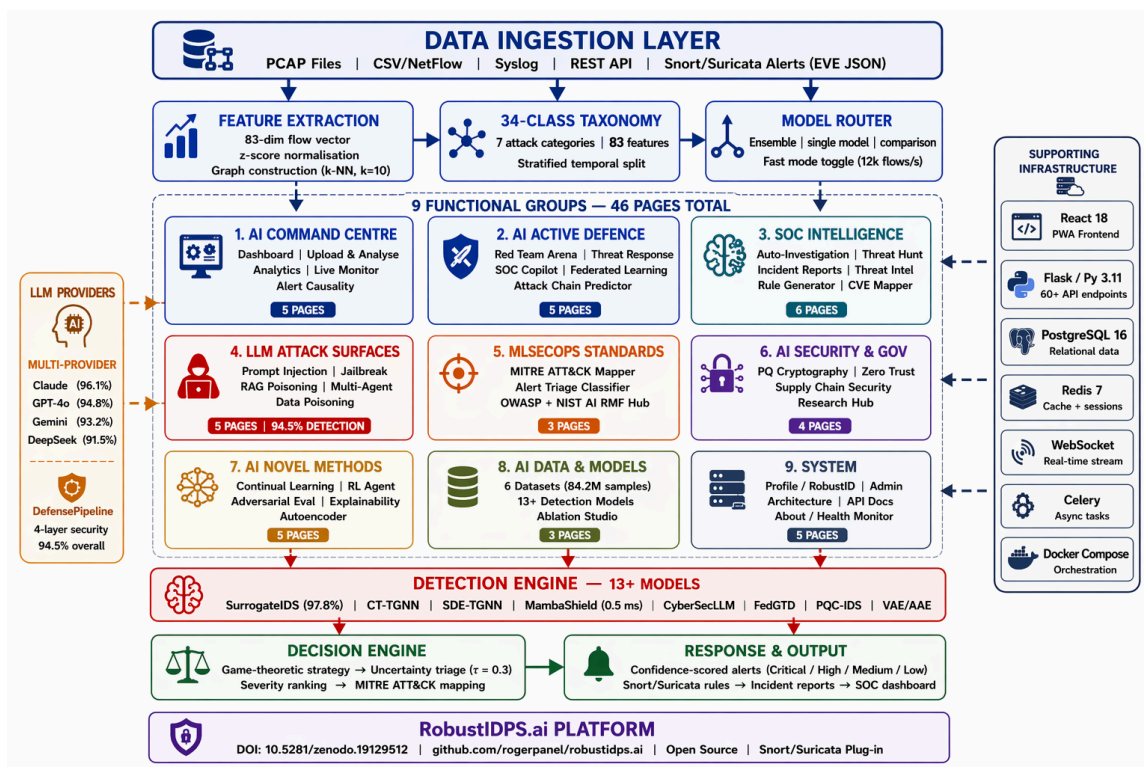
Рис. 5.1 – Высокоуровневая архитектура системы RobustIDPS.ai, показывающая все 9 функциональных групп, поддерживающую инфраструктуру (Docker Compose, PostgreSQL, Redis, WebSocket, Celery) и поток данных от приёма сырого трафика через обнаружение, анализ и реагирование.
