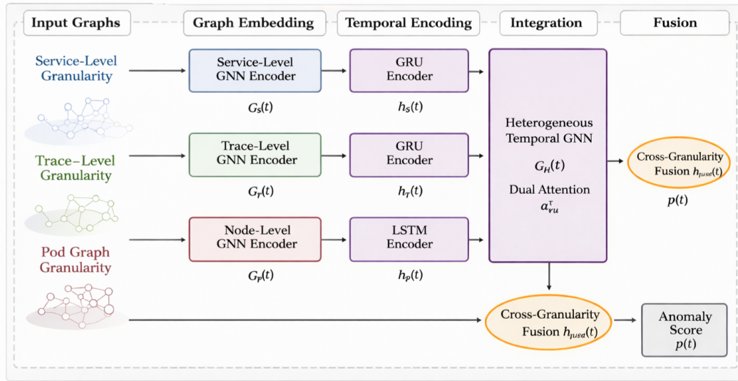
Рис. 2.3 – Принципиальная архитектура модели М3: TripleE-TGNN — тройного вложения для многоуровневого темпорального представления графов с двойным временно-пространственным вниманием и упругой консолидацией весов для предотвращения катастрофического забывания.
