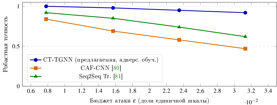
Рис. 6.5 – Зависимость робастной точности от бюджета PGD-атаки \varepsilon для трёх архитектур. Предлагаемая СТ-TGNN сохраняет робастную точность \geq 0,92 во всём исследуемом диапазоне.
