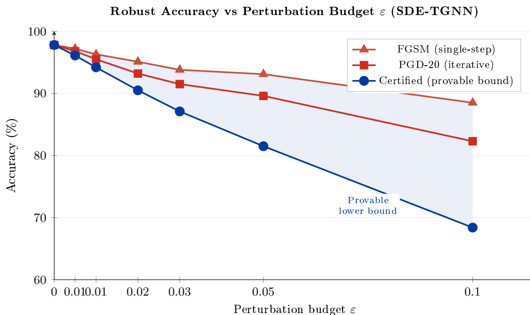
Рис. 4.6 – Робастная точность как функция бюджета возмущений \epsilon для FGSM, PGD-20 и сертифицированных (рандомизированное сглаживание) оценок SDE-TGNN. Сертифицированная кривая обеспечивает доказуемую нижнюю границу; FGSM и PGD представляют эмпирические верхние границы при конкретных стратегиях атак.
