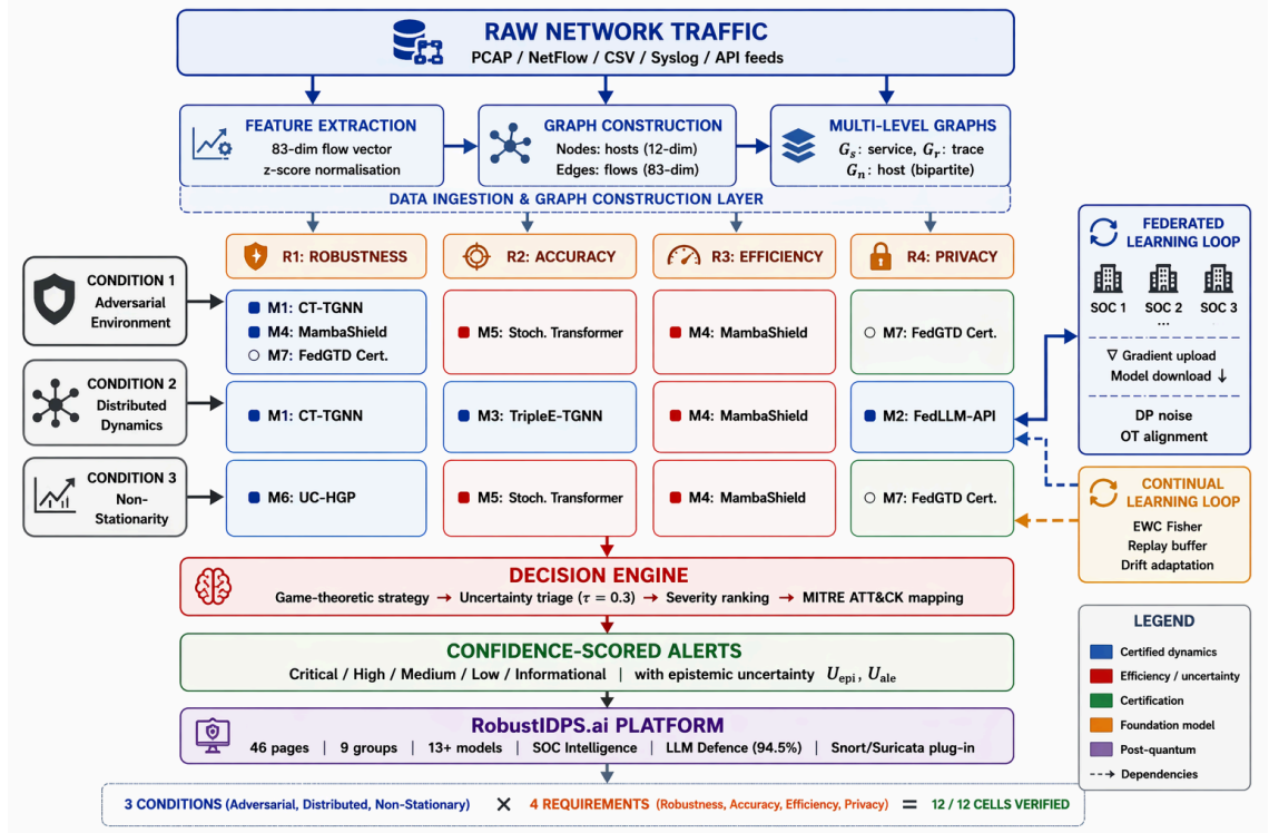
Рис. 3.6 – Интегрированный конвейер обнаружения, показывающий поток данных от сырого сетевого трафика через все семь методов к оповещениям, ранжированным по серьёзности и оценённым по уверенности. Модуль FedLLM-API синхронизирует модели через границы при дифференциальной приватности.
