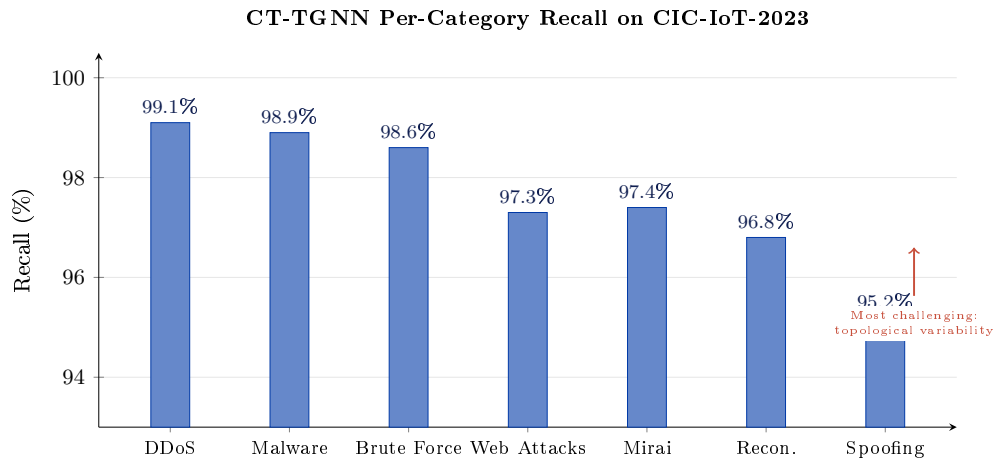
Рис. 3.13 – Покатегорийная полнота CT-TGNN на CIC-IoT-2023 по семи основным семействам атак. DDoS достигает наивысшей полноты (99,1%), тогда как спуфинг наиболее сложен (95,2%), что отражает его большую топологическую вариативность.
