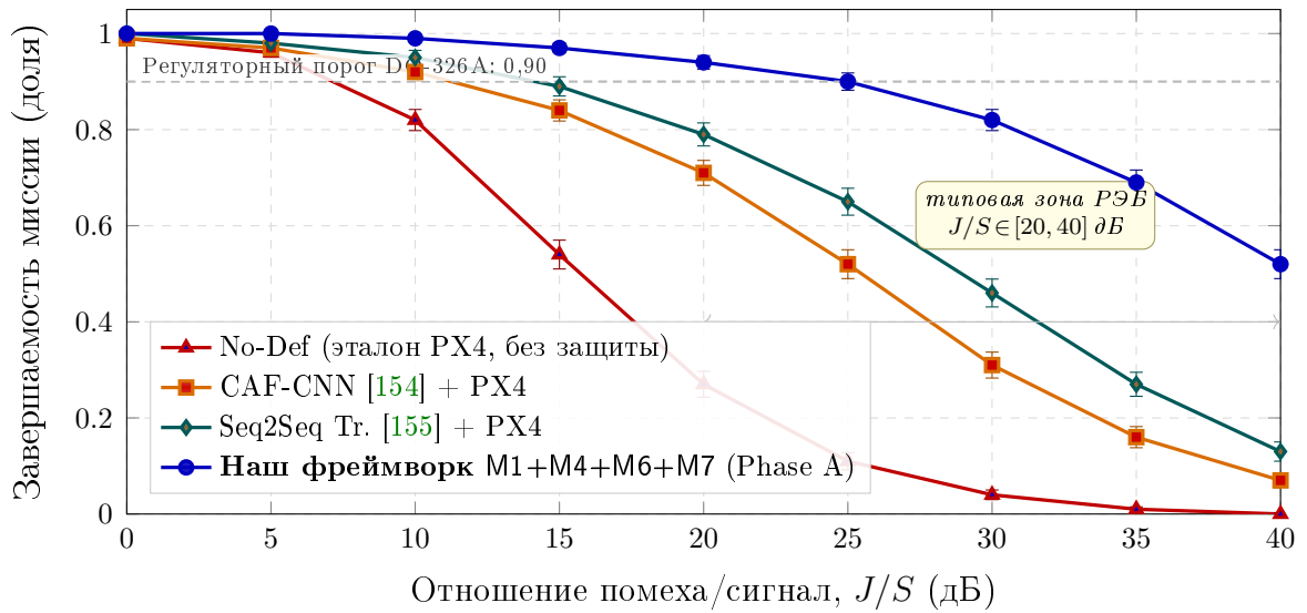
Рис. 6.6 – Завершаемость миссии БПЛА в зависимости от интенсивности РЭБ-подавления, измеренной как отношение мощности помехи к мощности полезного сигнала ( J/S , дБ). Эталон UAV-EW-Bench-2026: 5 000 симулированных вылетов (AirSim / PX4 SITL), три типа миссий, три модели ГНСС-приёмника, комбинированный состязательный контур. Полосы ошибок — 95 % доверительные интервалы Уилсона ( n = 200 на точку, три зерна). Предлагаемый фреймворк M1+M4+M6+M7 удерживает завершаемость выше регуляторного порога DO-326A 0,90 до J/S \approx 27 дБ включительно — против \approx 18 дБ для Seq2Seq Tr., \approx 13 дБ для CAF-CNN и \approx 7,5 дБ для эталонной PX4 без защиты, то есть выигрыш в 9–19 дБ по операционно-значимому показателю.
