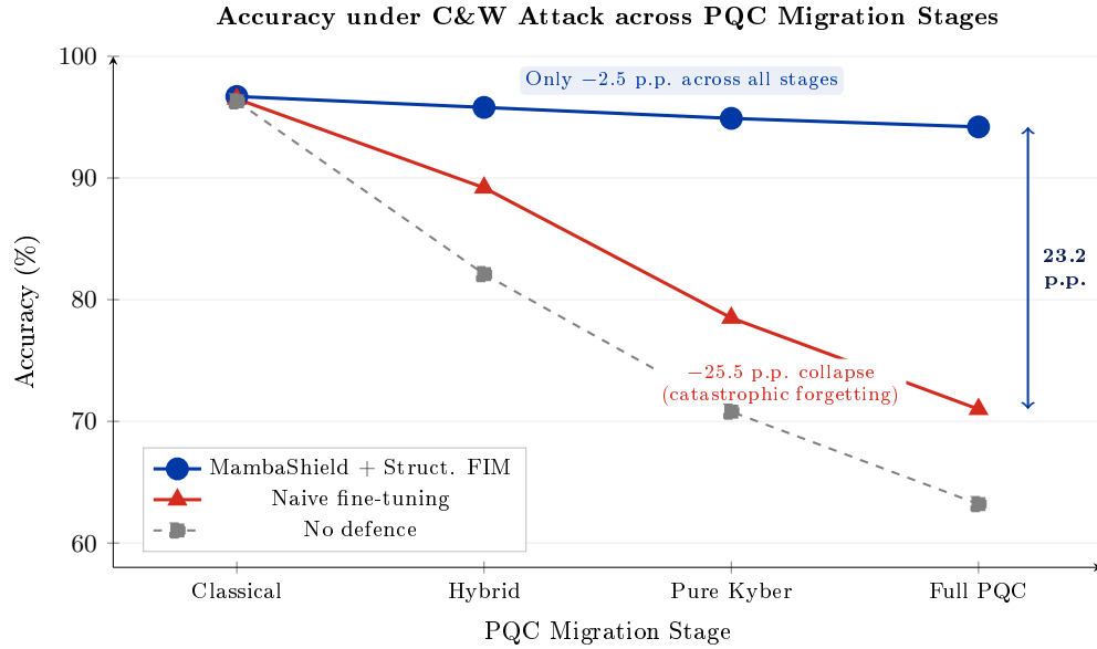
Рис. 4.8 – Точность при атаке C&W на четырёх этапах миграции PQC (Классический → Гибридный → Чистый Kyber → Полный PQC). MambaShield со структурированной FIM сохраняет точность в пределах 2,5 п. п. на всех этапах, тогда как наивное дообучение обрушивается на 25,5 п. п. из-за катастрофического забывания классических паттернов трафика.
