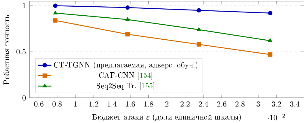
Рис. 6.4 – Зависимость робастной точности от бюджета PGD-атаки \epsilon для трёх архитектур. Предлагаемая СТ-TGNN сохраняет робастную точность \geq 0,92 во всём исследуемом диапазоне.
