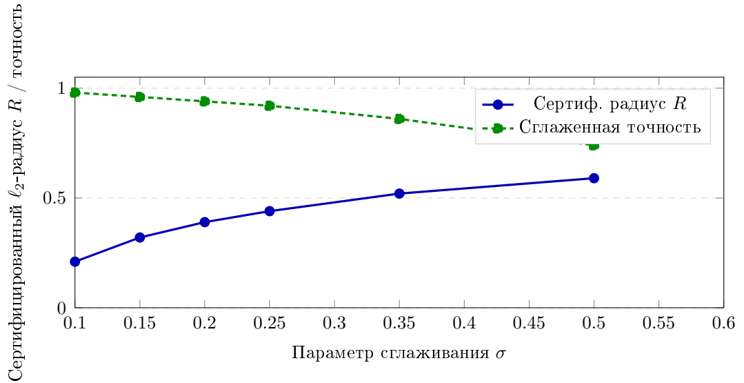
Рис. 6.5 – Компромисс между параметром сглаживания \sigma , сертифицированным \ell_2 -радиусом и точностью сглаженного классификатора (Cohen-style, \alpha = 10^{-3} ).
