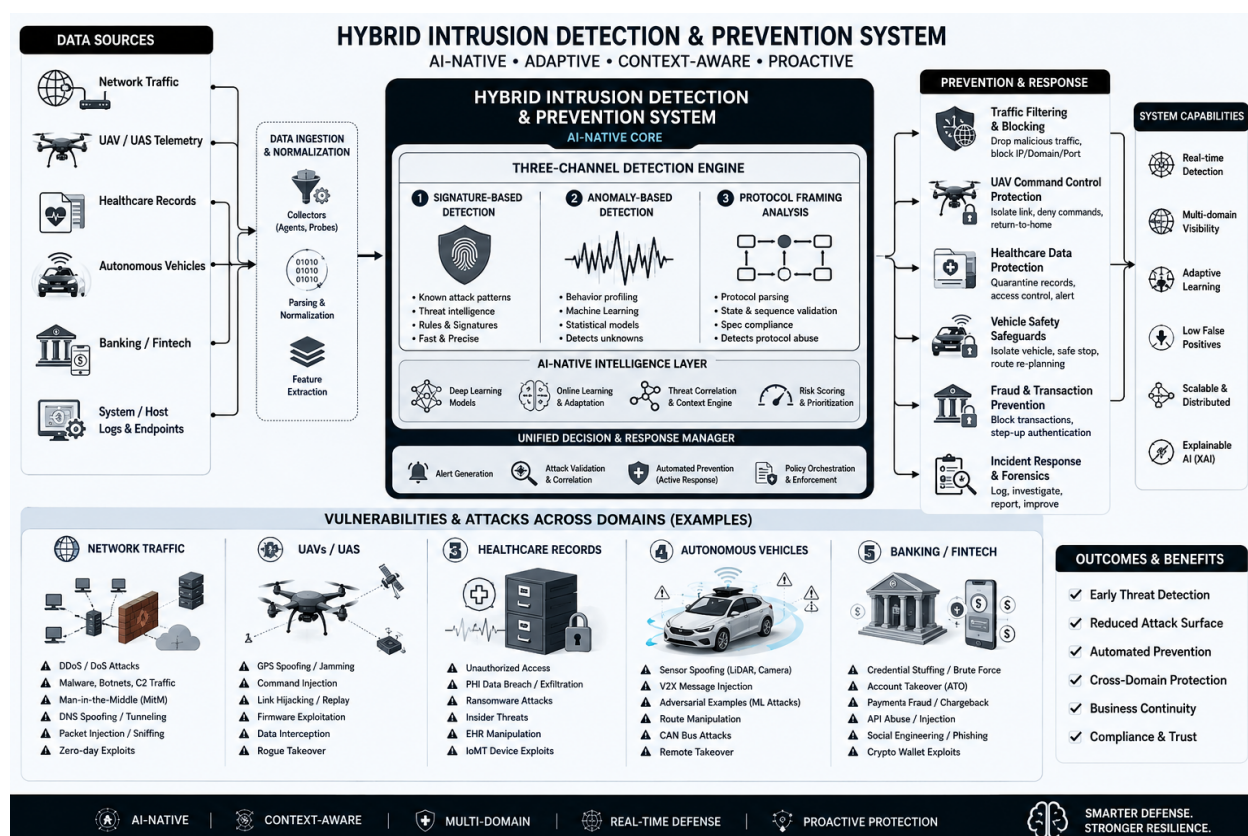
Рис. 1.1 – Интегрированная схема гибридной СОПВ: AI-нативное, адаптивное, контекстно-зависимое, упреждающее защитное решение. Слева — источники данных (сетевой трафик, телеметрия БПЛА, медицинские записи, автономные транспортные средства, банковский/финтех-трафик, системные журналы); по центру — ядро системы с трёхканальным детектированием (сигнатурное, аномалийное, протокольный анализ), AI-нативным интеллектуальным слоем (глубокое обучение, онлайн-обучение, корреляция угроз, оценка риска) и единым менеджером решений и реагирования; справа — блок предотвращения и реагирования (фильтрация трафика, защита команд БПЛА, защита медицинских данных, активная безопасность транспортных средств, предотвращение мошенничества, инцидент-форензика) и системные возможности (обнаружение в реальном времени, многосекторная видимость, адаптивное обучение, низкая доля ложных срабатываний, масштабируемость, объяснимый ИИ). Нижняя панель приводит характерные классы уязвимостей в каждом из пяти показательных секторов.
