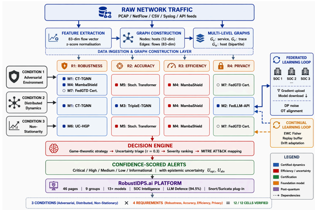
Рис. 3.11 – Интегрированный конвейер обнаружения, показывающий поток данных от сырого сетевого трафика через все семь методов к оповещениям, ранжированным по серьёзности и оценённым по уверенности. Модуль FedLLM-API синхронизирует модели через границы при дифференциальной приватности.
