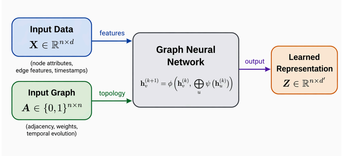
Рис. 2 – Двойственная природа входов ГНС-моделей, применяемых в качестве одной из ветвей обучаемых детекторов в системах гибридная СОПВ. Модель одновременно получает числовые данные (матрица признаков \mathbf{X} ) и реляционную структуру (матрица смежности \mathbf{A} ). Возмущение любого из входов может нарушить обученное представление, что мотивирует разработку системы повышения робастности и эффективности гибридная СОПВ, являющейся предметом настоящей диссертации.
