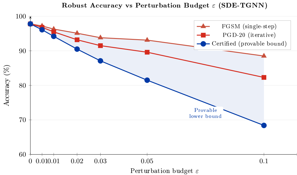
Рис. 4.6 – Робастная точность как функция бюджета возмущений \varepsilon для FGSM, PGD-20 и сертифицированных (рандомизированное сглаживание) оценок SDE-TGNN. Сертифицированная кривая обеспечивает доказуемую нижнюю границу; FGSM и PGD представляют эмпирические верхние границы при конкретных стратегиях атак.
