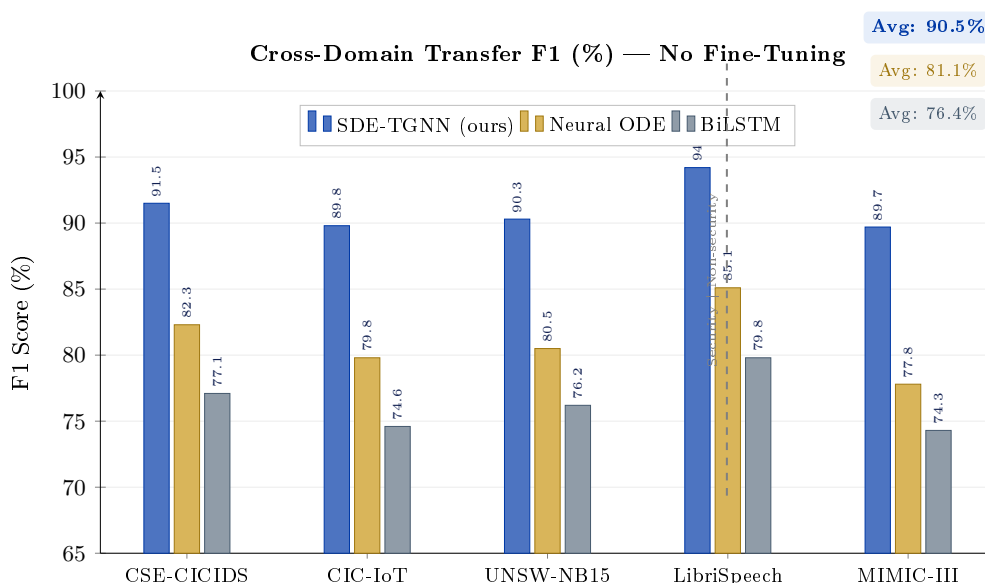
Рис. 4.7 – Кросс-доменный перенос F1 (%) для SDE-TGNN, базовой линии Neural ODE и базовой линии BiLSTM на трёх наборах данных безопасности и двух областях вне безопасности (речь, здравоохранение). SDE-TGNN достигает 90,5% среднего переноса без дообучения, что на 9,4 п. п. выше Neural ODE и на 14,1 п. п. выше BiLSTM.
