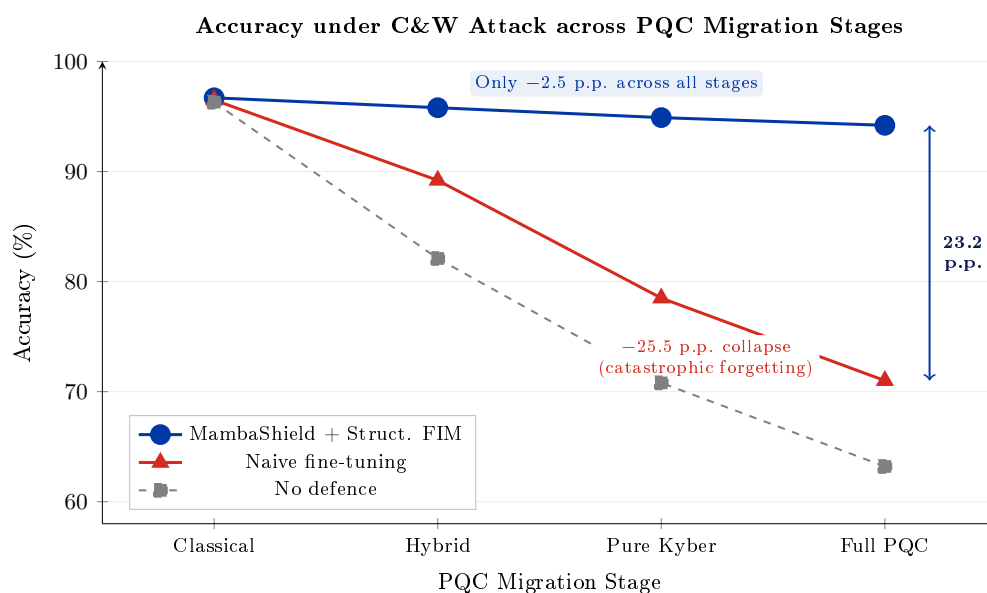
Рис. 4.9 – Точность при атаке C&W на четырёх этапах миграции PQC (Классический → Гибридный → Чистый Kyber → Полный PQC). MambaShield со структурированной FIM сохраняет точность в пределах 2,5 п. п. на всех этапах, тогда как наивное дообучение обрушивается на 25,5 п. п. из-за катастрофического забывания классических паттернов трафика.
