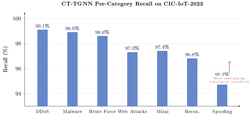
Рис. 4.2 – Покатегорийная полнота СТ-TGNN на CIC-IoT-2023 по семи основным семействам атак. DDoS достигает наивысшей полноты (99,1%), тогда как спуфинг наиболее сложен (95,2%), что отражает его большую топологическую вариативность.
