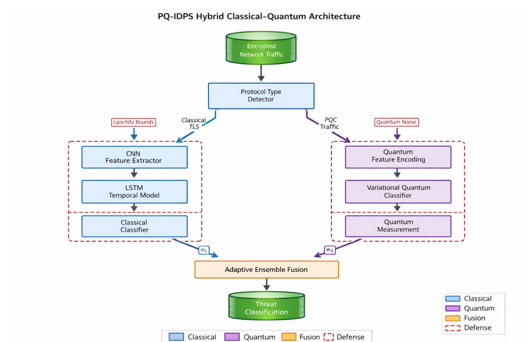
Рис. 3.7 – Прямо совместимая мультипротокольная архитектура обнаружения для постквантового трафика.
