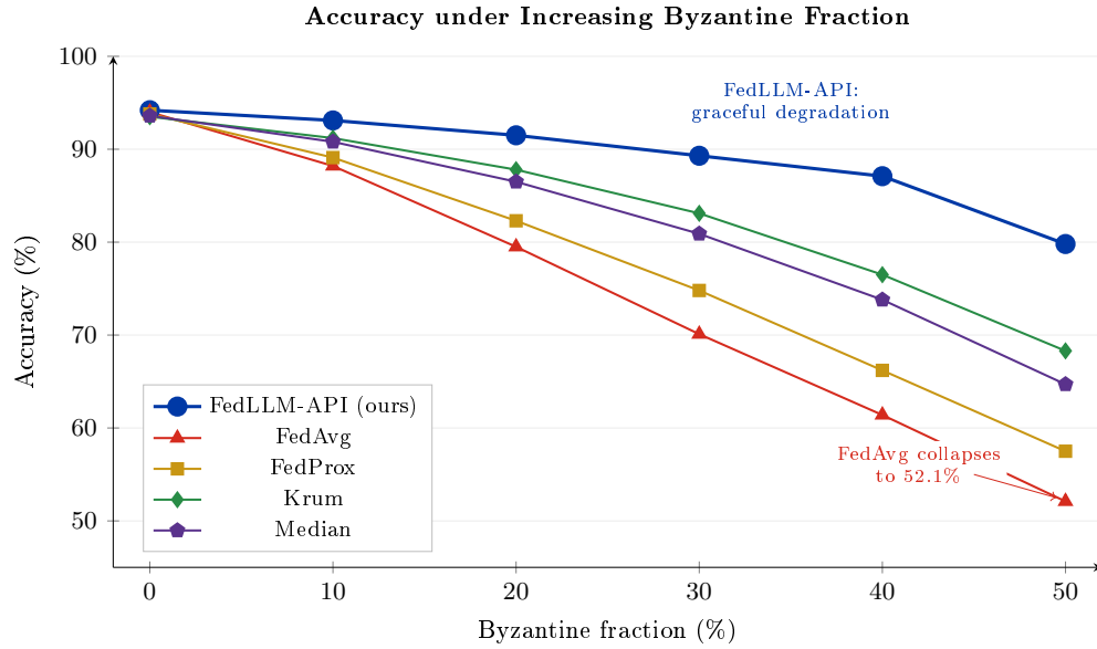
Рис. 4.4 – Деградация точности FedLLM-API при увеличении доли византийских участников в сравнении с базовыми линиями FedAvg, FedProx, Krum и Медиана. FedLLM-API плавно деградирует с 94,2% до 79,8% при увеличении повреждения с 0% до 50%, тогда как FedAvg обрушивается до 52,1%.
