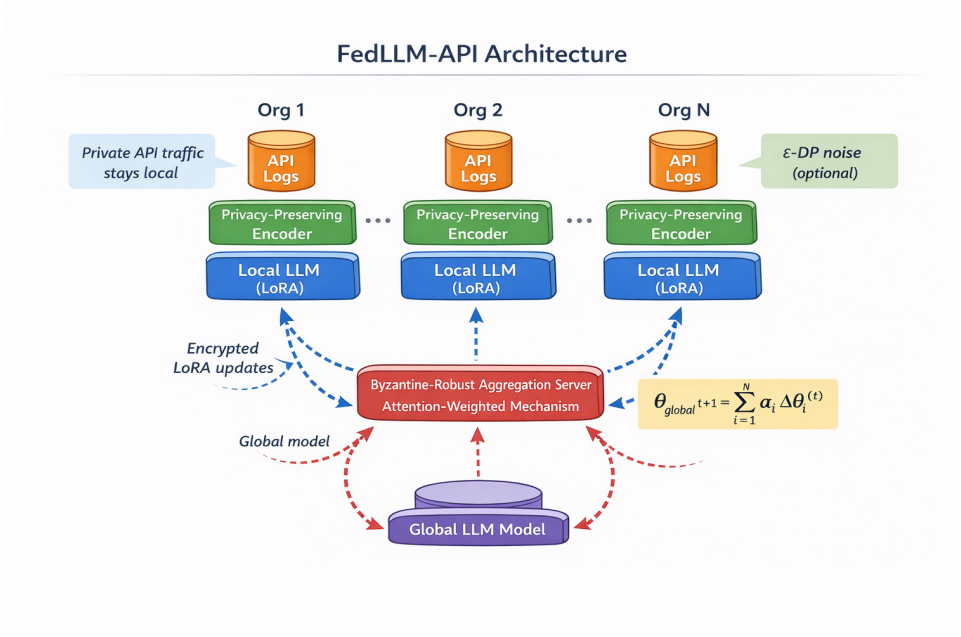
Рис. 3.2 – Архитектура FedLLM-API для совместной разведки угроз через организационные границы.
