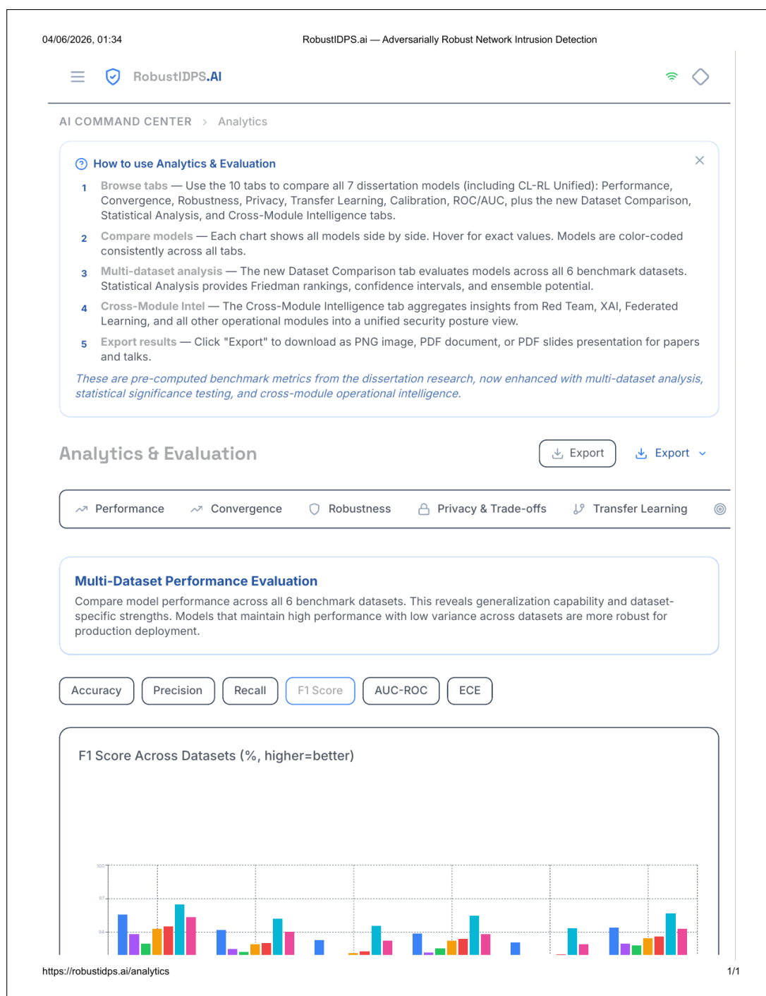
Рис. 3.10 – Страница Analytics & Evaluation с подсказкой «Как пользоваться»: интерактивные пояснения к десяти вкладкам сравнительной оценки моделей, экспорт результатов в PNG/PDF и PDF-презентацию.
