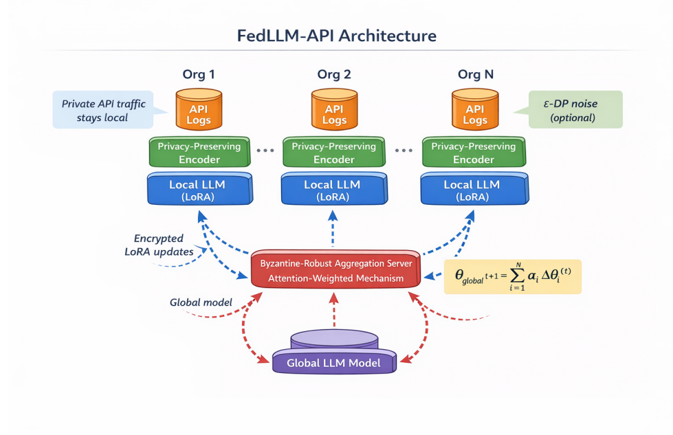
Рис. 3.2 – Архитектура FedLLM-API для совместной разведки угроз через организационные границы.
