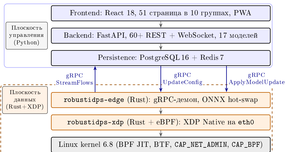
Рис. 5.3 – Двухплоскостная архитектура RobustIDPS.ai v4: Python-плоскость управления (синяя рамка, верх) и Rust-плоскость данных (оранжевая пунктирная рамка, низ) разделены чёткой границей и связаны тремя gRPC-примитивами. StreamFlows — поток записей о потоках из плоскости данных в плоскость управления; UpdateConfig — проталкивание списков блокировки в обратном направлении; ApplyModelUpdate — атомарная доставка INT8 ONNX-ученика на работающие агенты без перезапуска.
