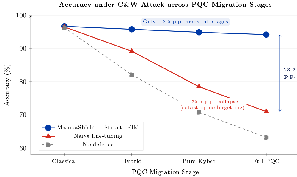
Рис. 4.9 – Точность при атаке C&W на четырёх этапах миграции PQС (Классический → Гибридный → Чистый Kyber → Полный PQС). MambaShield со структурированной FIM сохраняет точность в пределах 2,5 п. п. на всех этапах, тогда как наивное дообучение обрушивается на 25,5 п. п. из-за катастрофического забывания классических паттернов трафика.
