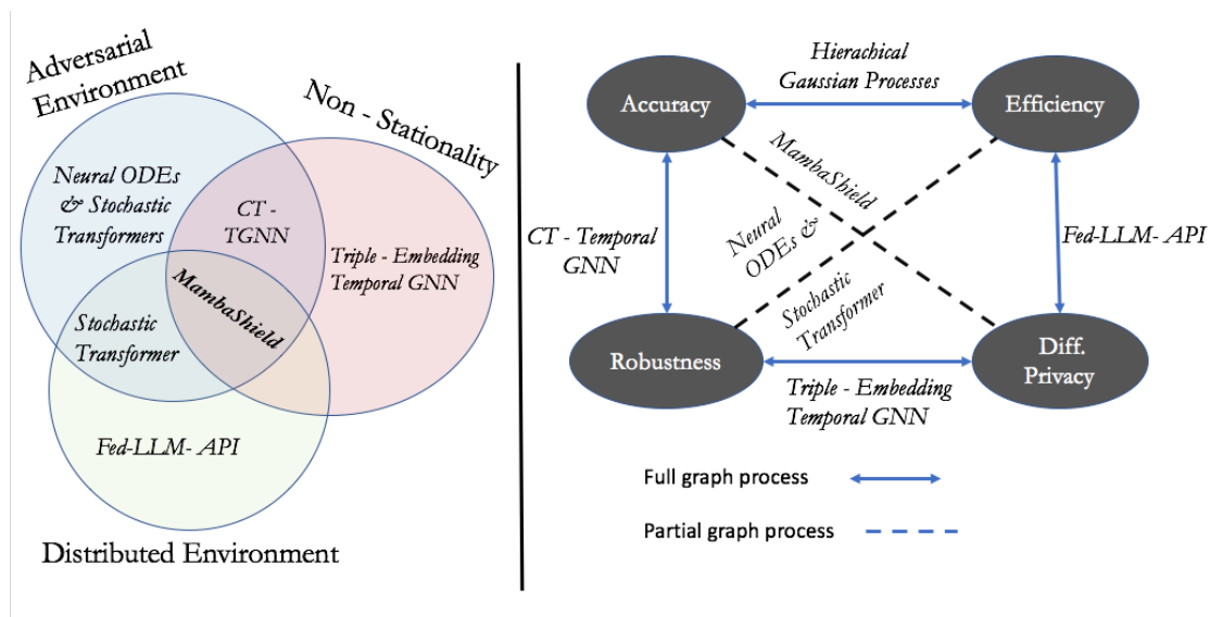
Рис. 3 – Расположение семи методов в пространстве условий функционирования (слева) и требований (справа). М4: MambaShield находится на пересечении всех трёх условий; М1: CT-TGNN связывает состязательное и нестационарное условия через сертифицированные непрерывно-временные динамики.
