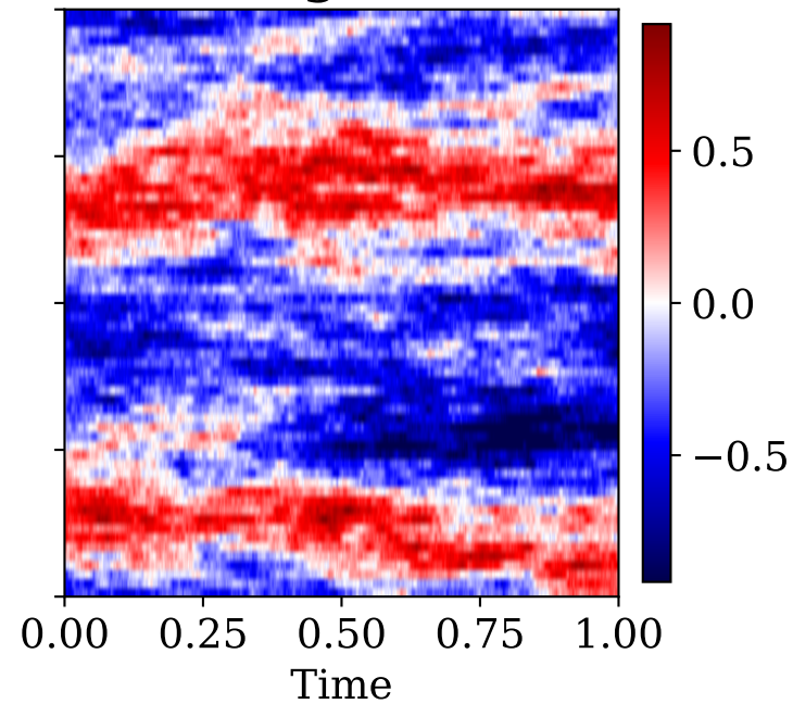
Nagumo
