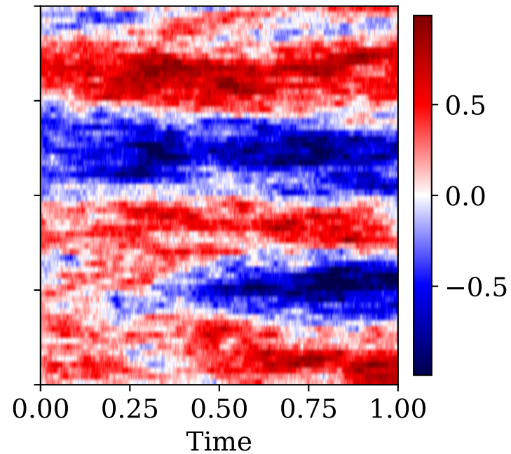
Allen-Cahn
