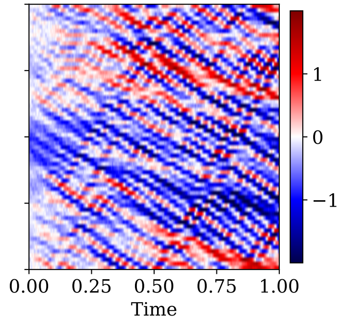
KdV
