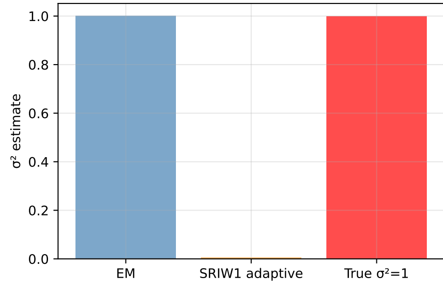
KM diffusion estimate
