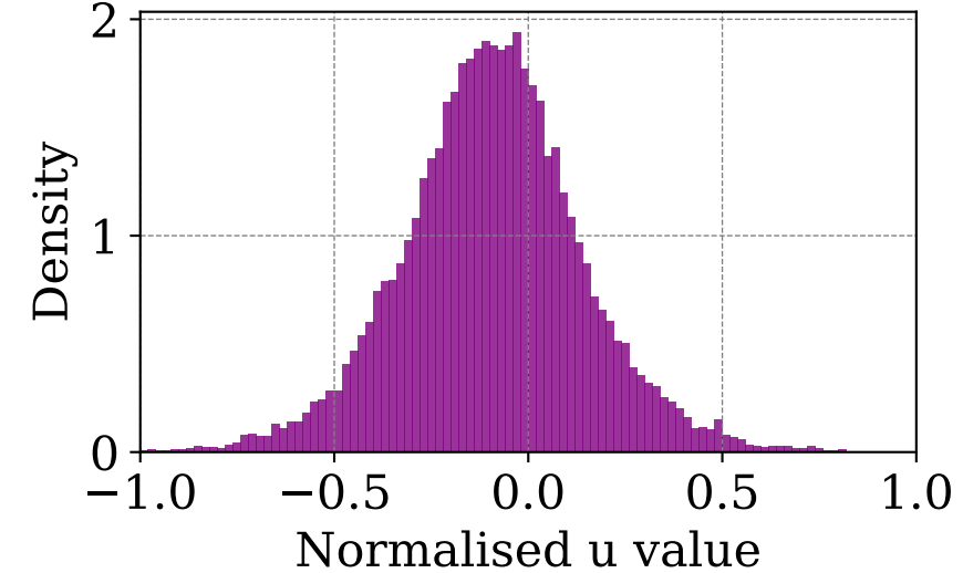
KdV
