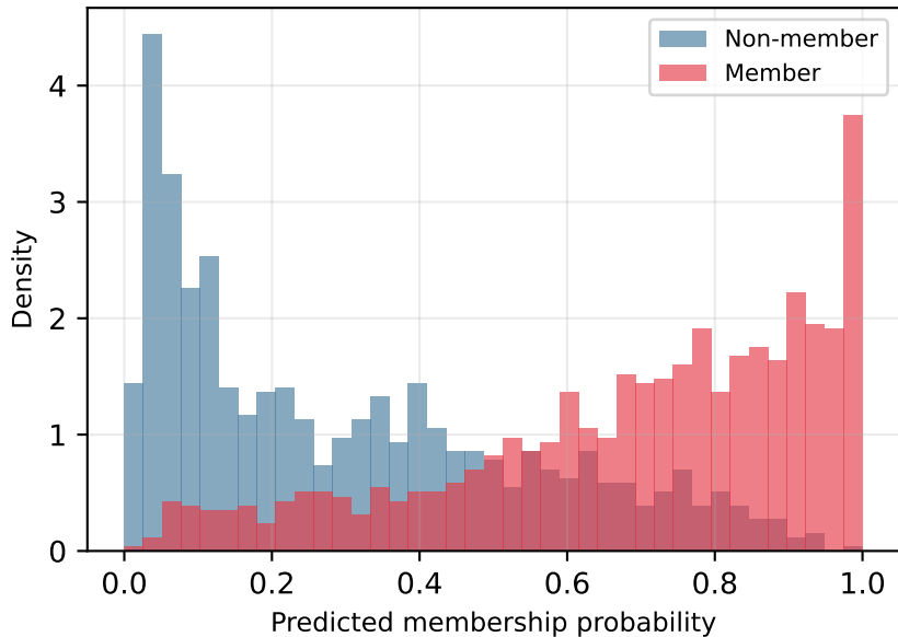
XGBoost (AUC=0.8559)
