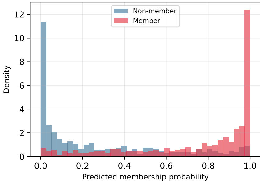
MLP (AUC=0.8544)
