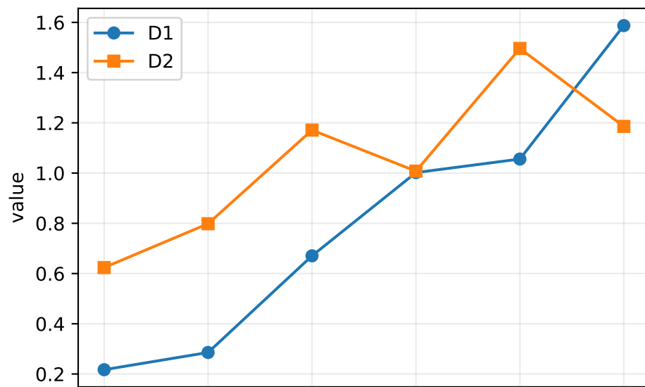
NLL
