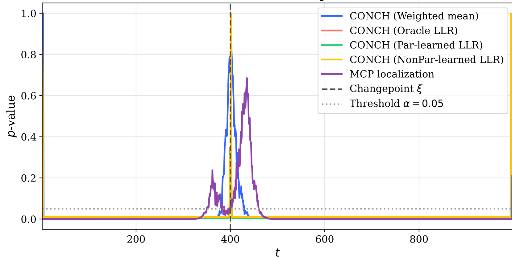
Gaussian mean shift p-values
