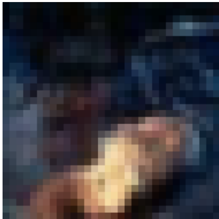
t=401 cls=4
