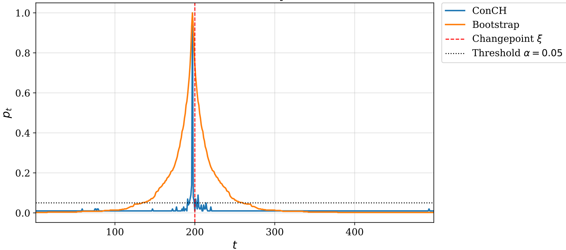
P-values (overlay)
