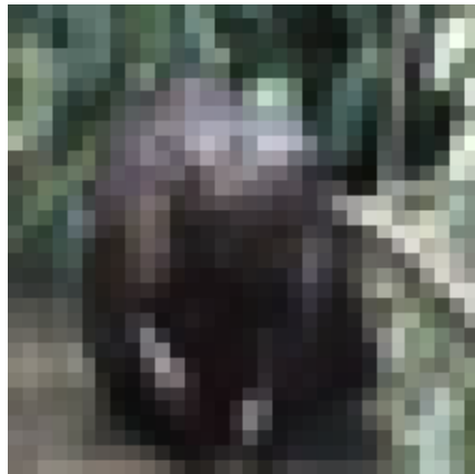
t=402 cls=4
