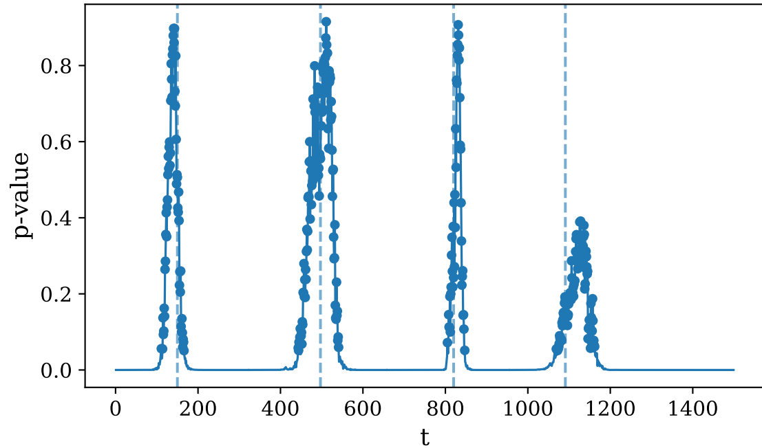
p-values
