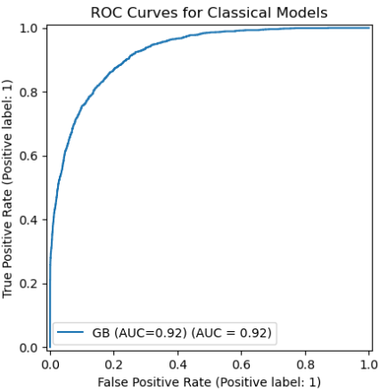
Tabular ROC Curves
