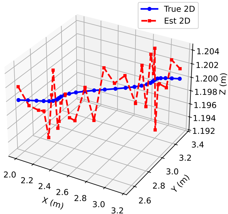
2D Tracking (Z constrained)
