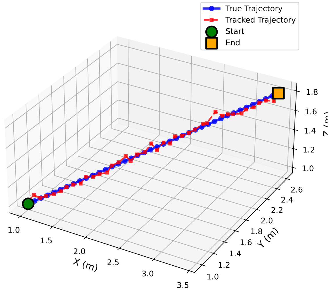
Linear Movement Mean Error: 0.03cm, Max: 0.10cm
