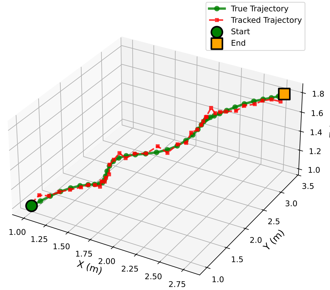
Zigzag Movement Mean Error: 0.03cm, Max: 0.10cm
