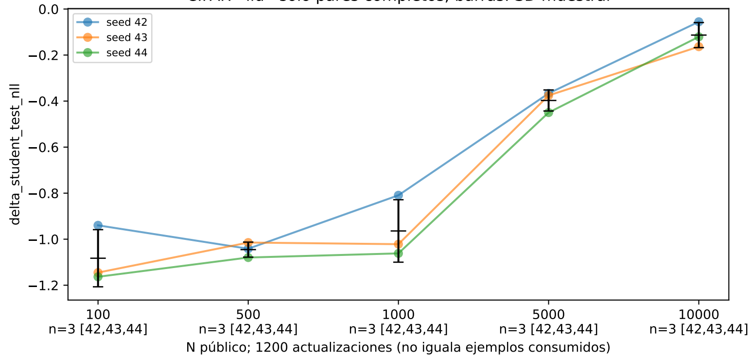
CIFAR · iid · solo pares completos; barras: SD muestral
