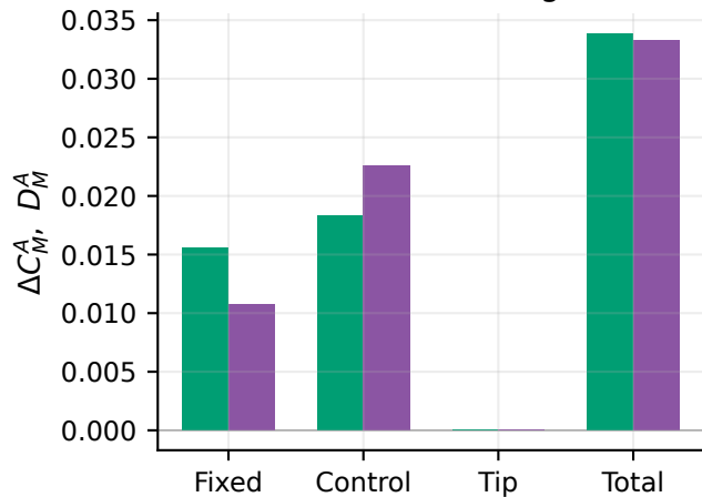
(d) Moment changes
