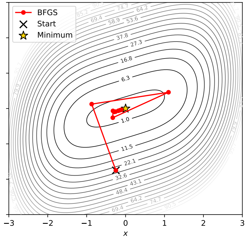
BFGS
