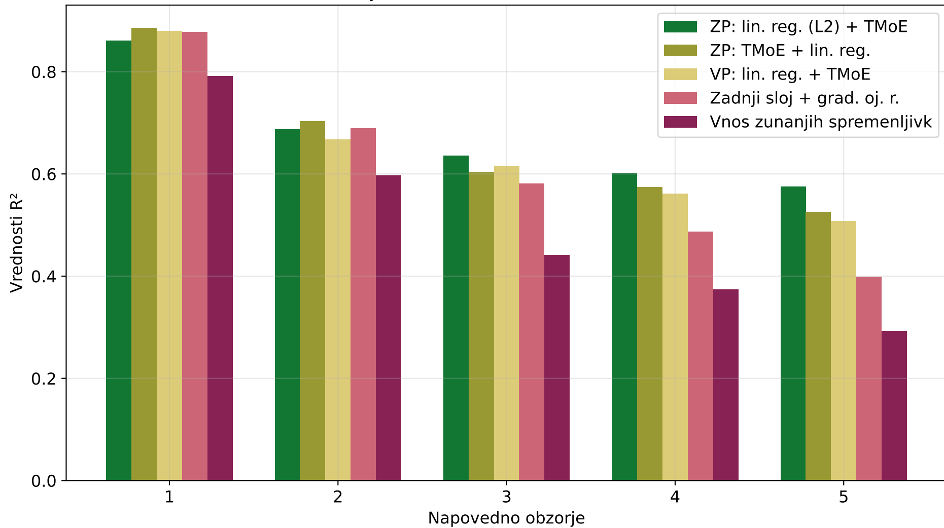
Primerjava metod za razširitev Time-MoE
