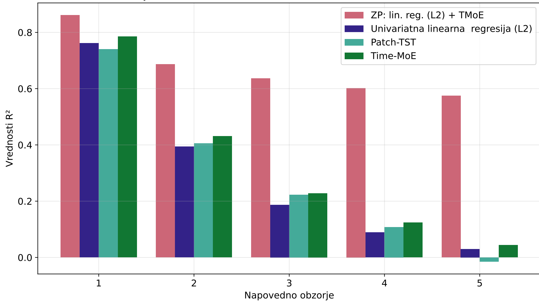
Primerjava metod za razširitev Time-MoE in univariatnih modelov
