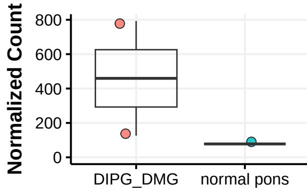
CCL2
