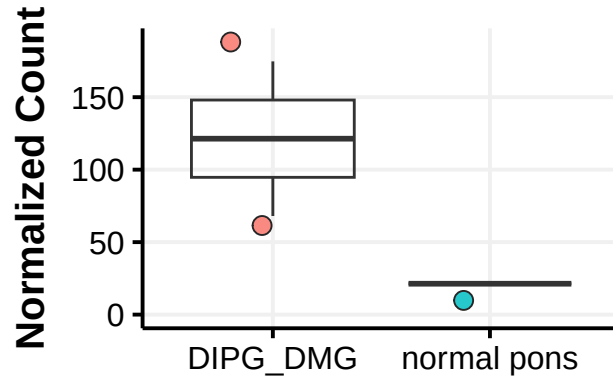
PTGS2
