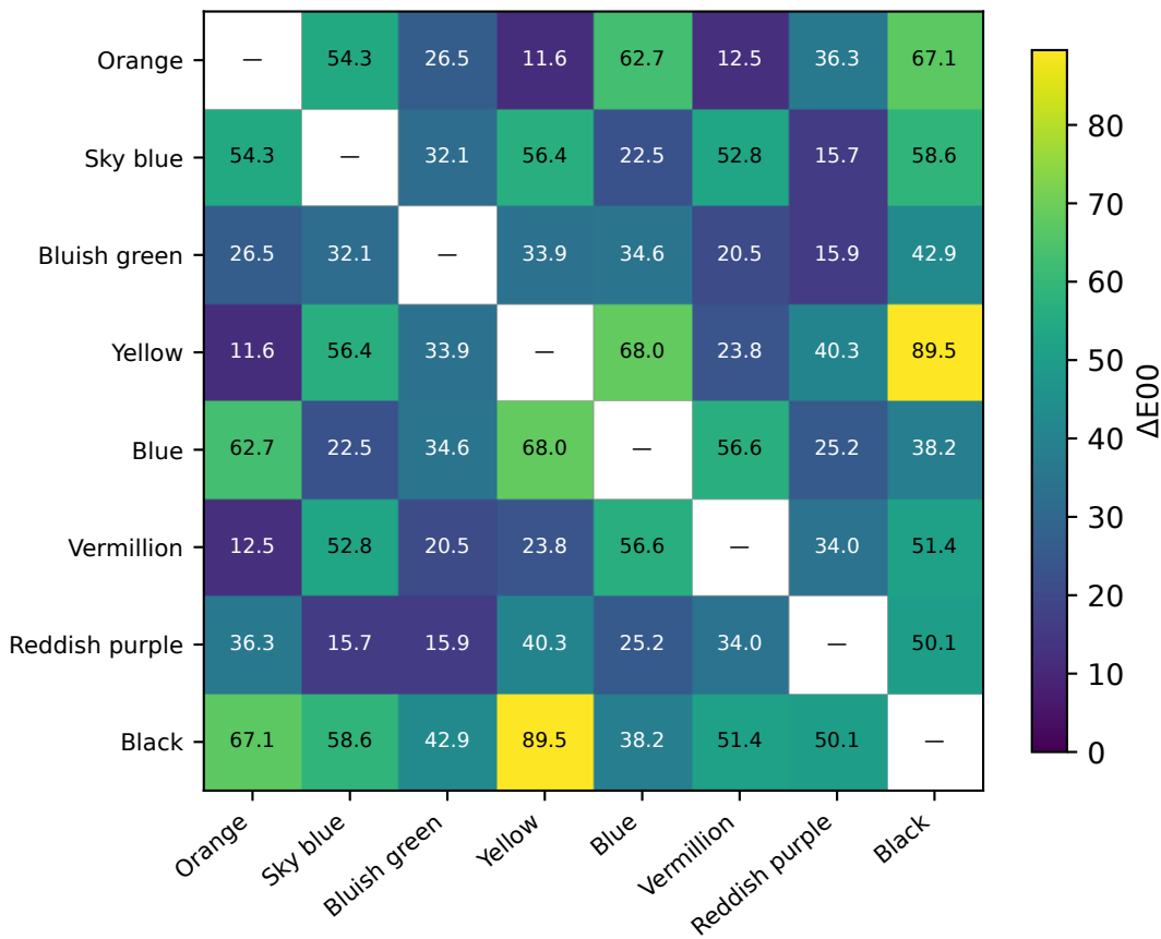
CIEDE2000 — Deutan 100%
