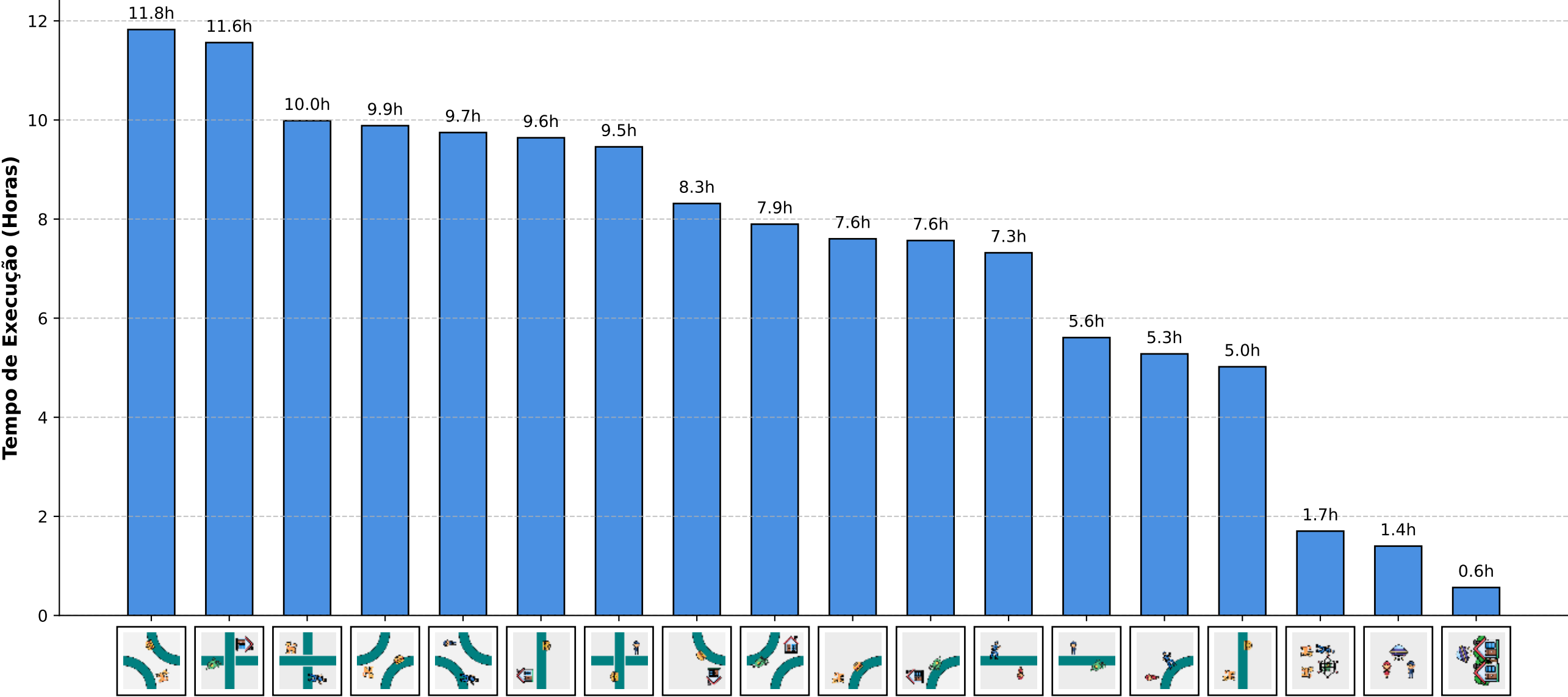
Tempo de Execução das Subárvores de Busca
