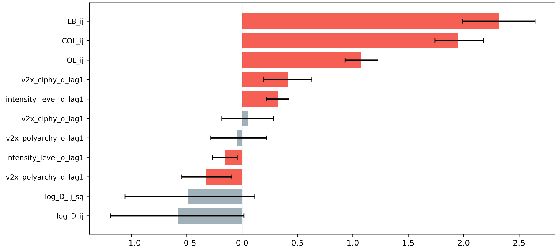
Coefficients Gravité — 50 pays (IC 90%) Rouge = IC excludant 0
