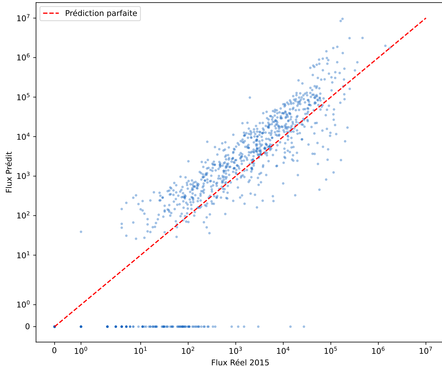
OOS 2015 — Observé vs Prédit (33 pays, MAE = 48,434)
