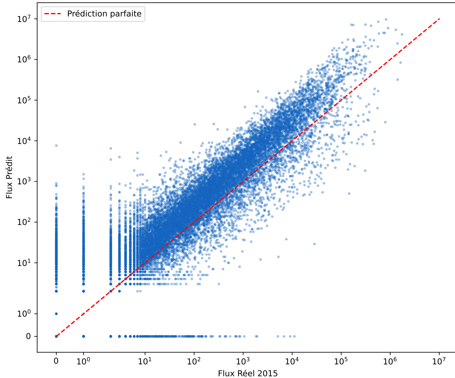
OOS 2015 — Observé vs Prédit (190 pays, MAE = 8,814)
