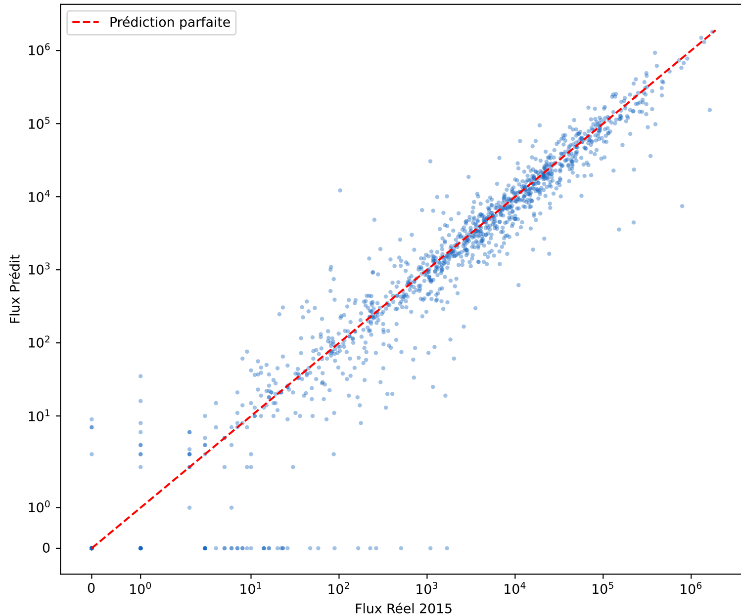
OOS 2015 — Observé vs Prédit (35 pays, MAE = 11,796)
