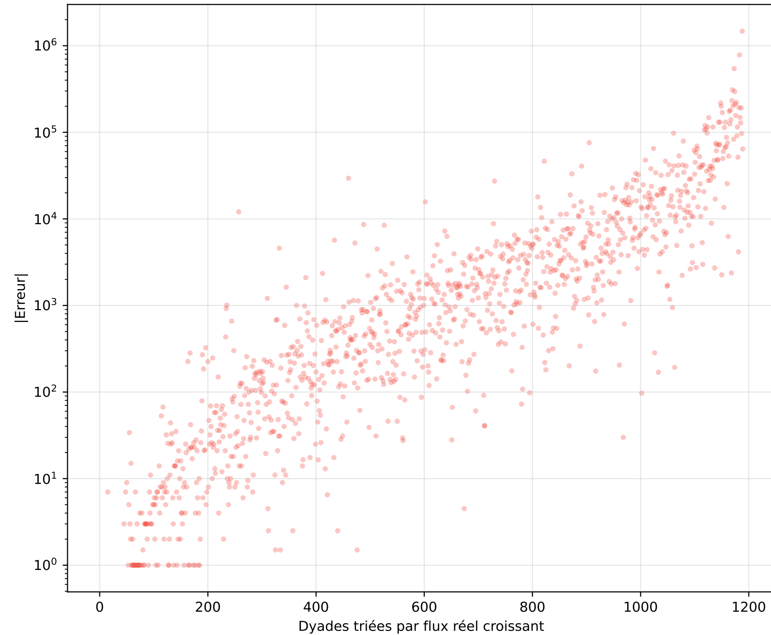
Distribution des erreurs absolues — 35 pays
