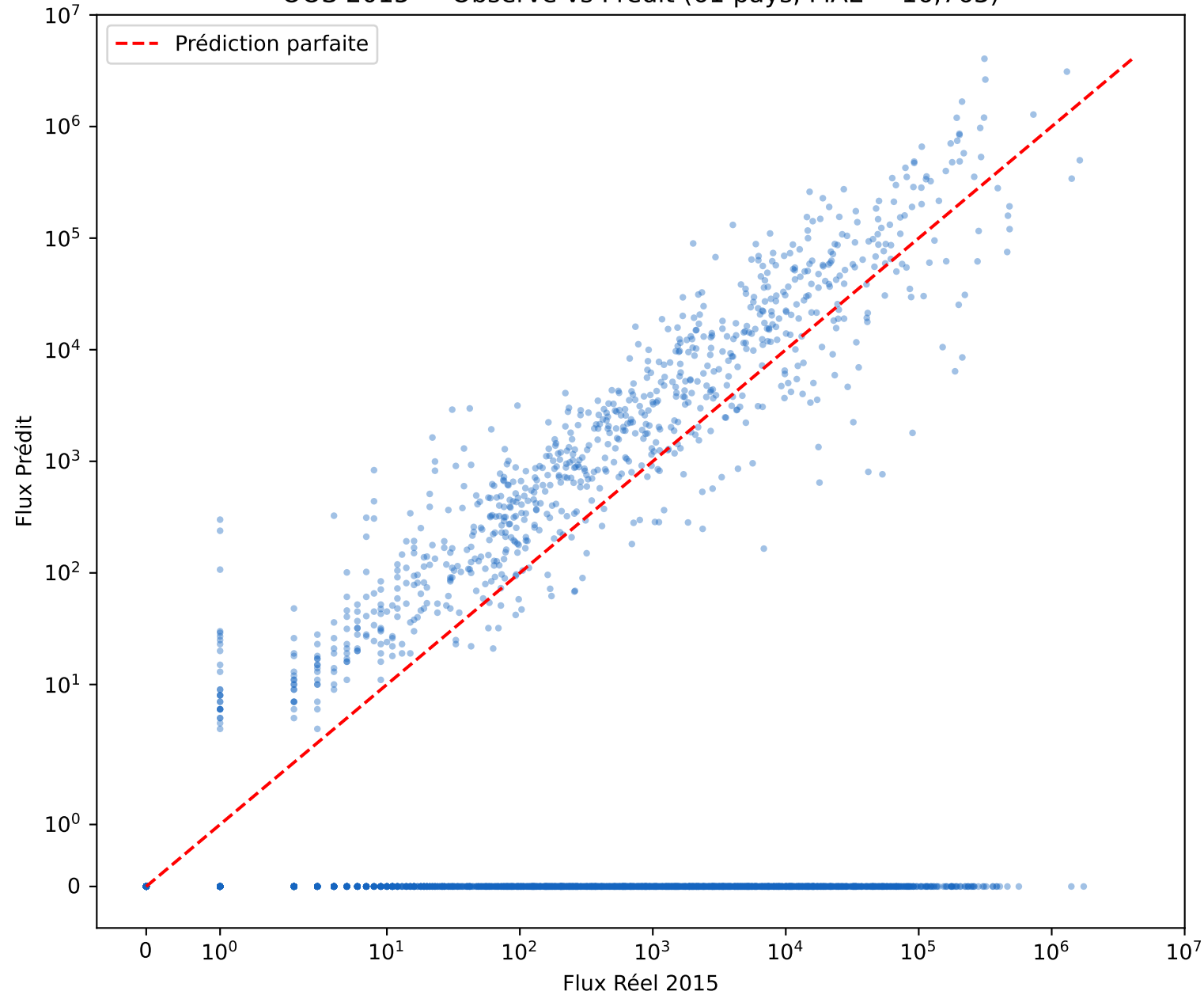
OOS 2015 — Observé vs Prédit (61 pays, MAE = 16,763)
