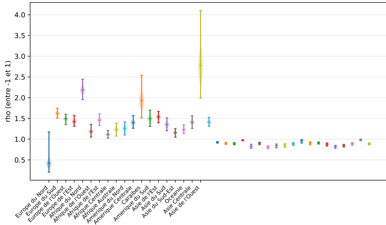
Inertie AR(1) par cluster M49
