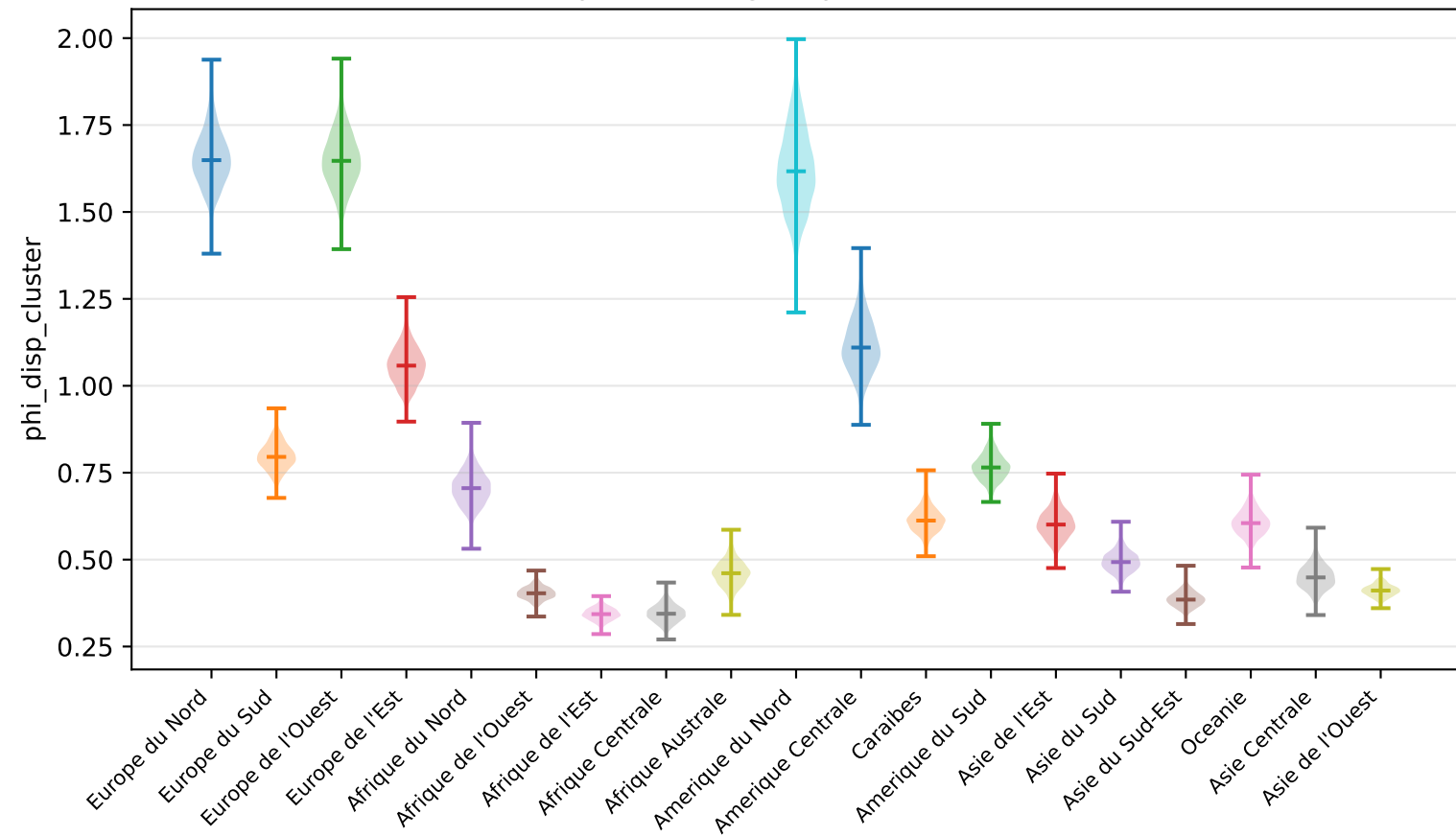
Dispersion NegBin par cluster M49
