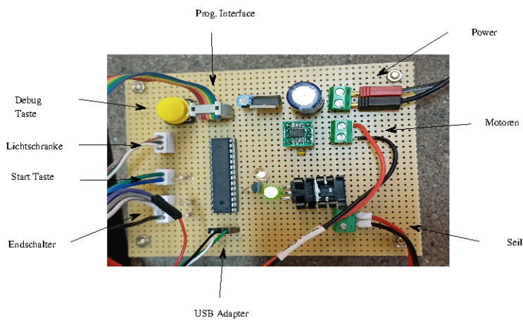
Abbildung 2: Anschlüsse der neuen Steuerung
