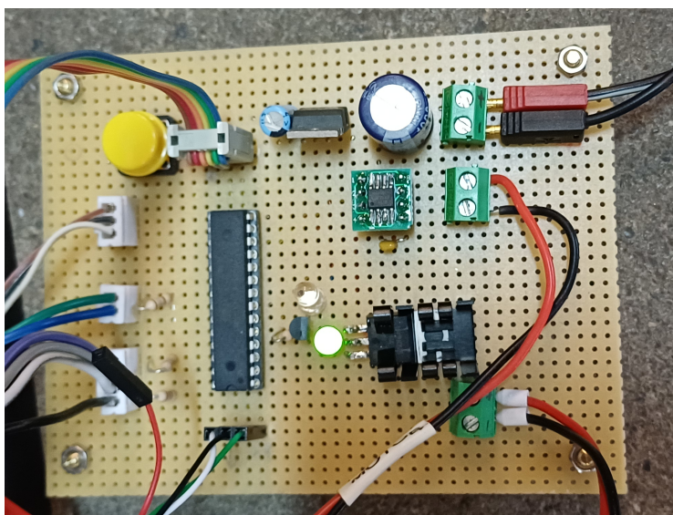
Abbildung 3: Anschlüsse der alten Steuerung
