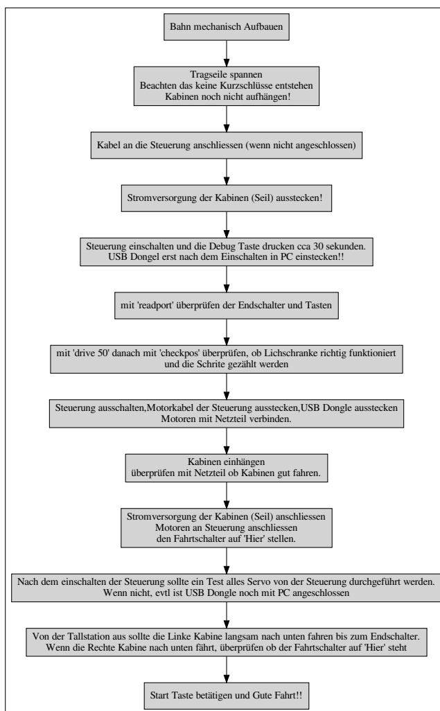
Abbildung 1: Ablauf der Installation, folgend Details zu der Installation
