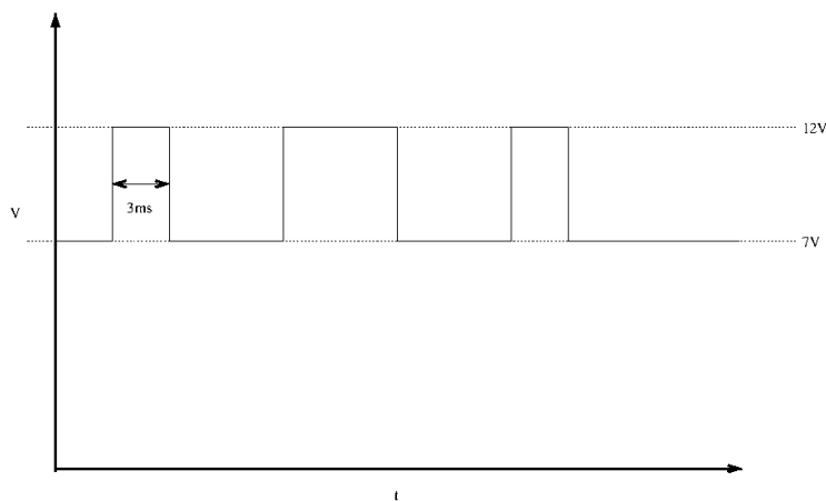
Abbildung 6: Seriale Übertragung zu den Kabinen und Tower
