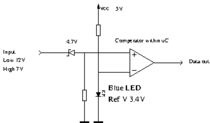
Abbildung 7: Funktionsweise der Detektierung
