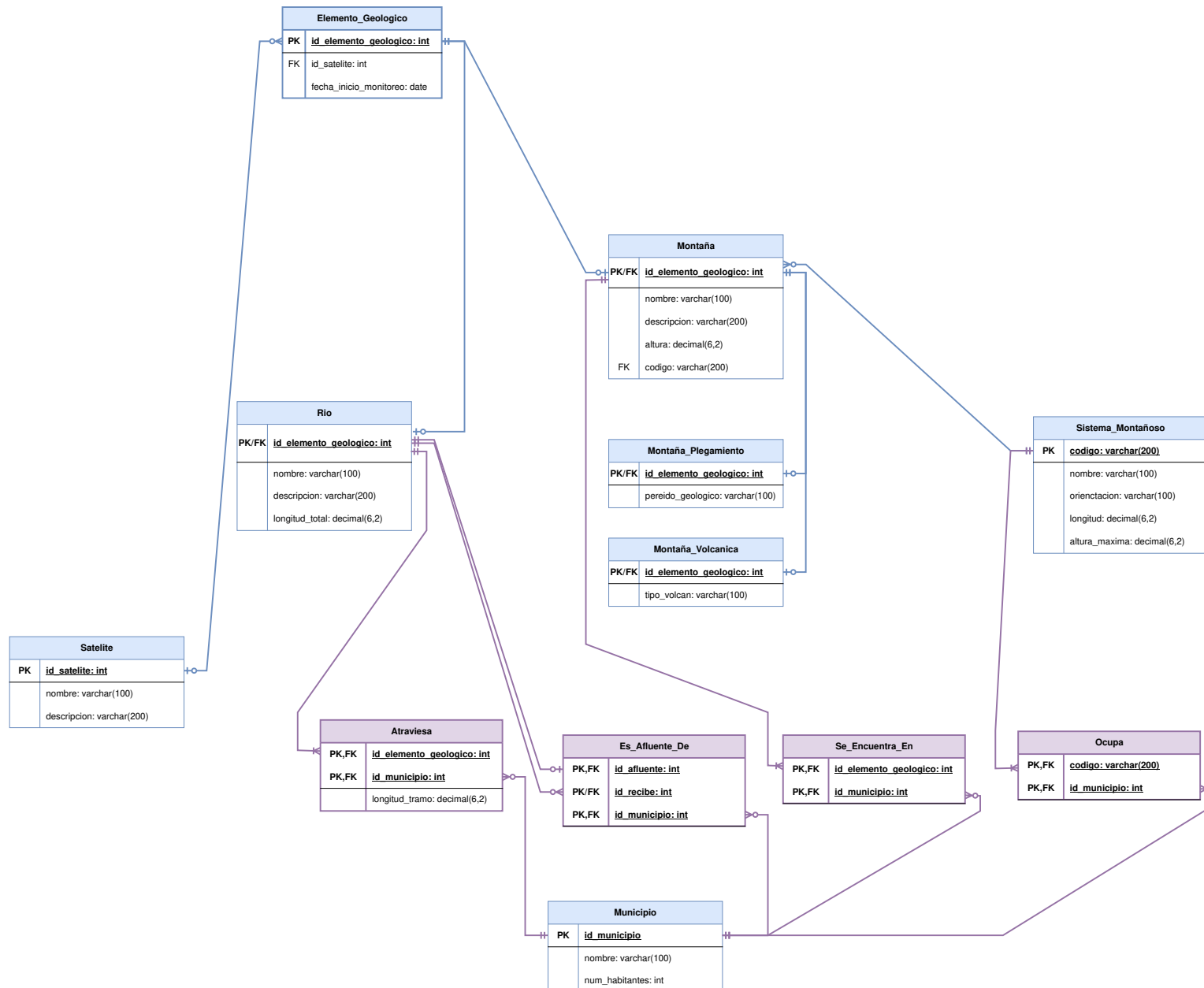
Figura 4: Modelo Racional para Sistema de Informacion Geografica.
