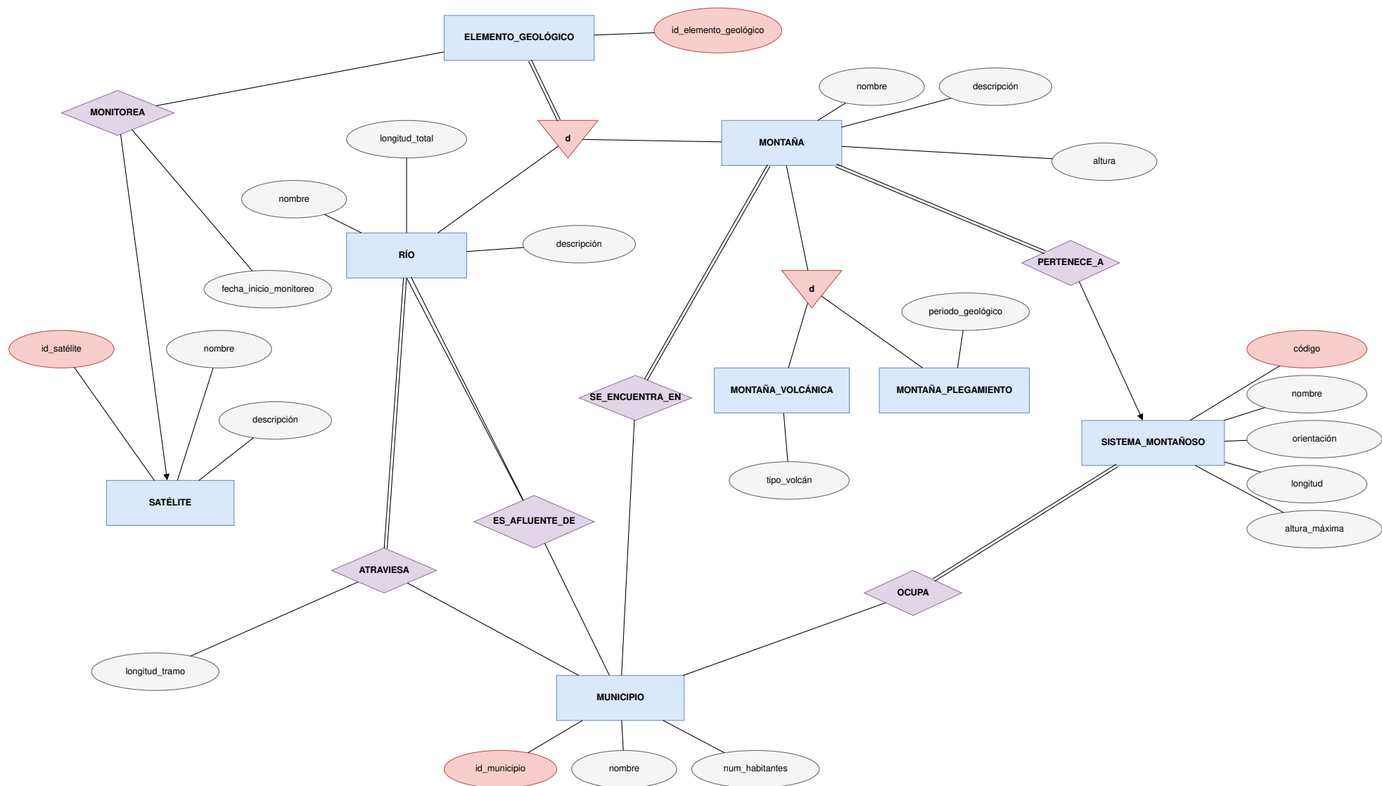
Figura 3: Modelo E-R para Sistema de Informacion Geografica.
