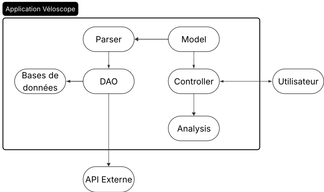
FIGURE 2 : Diagramme d'architecture
