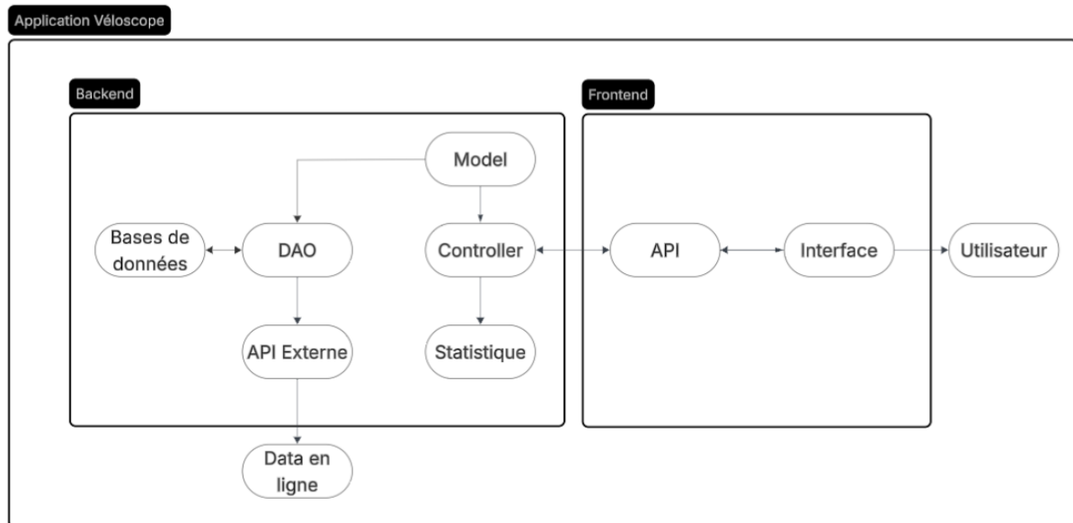
FIGURE 2 : Diagramme d'architecture
