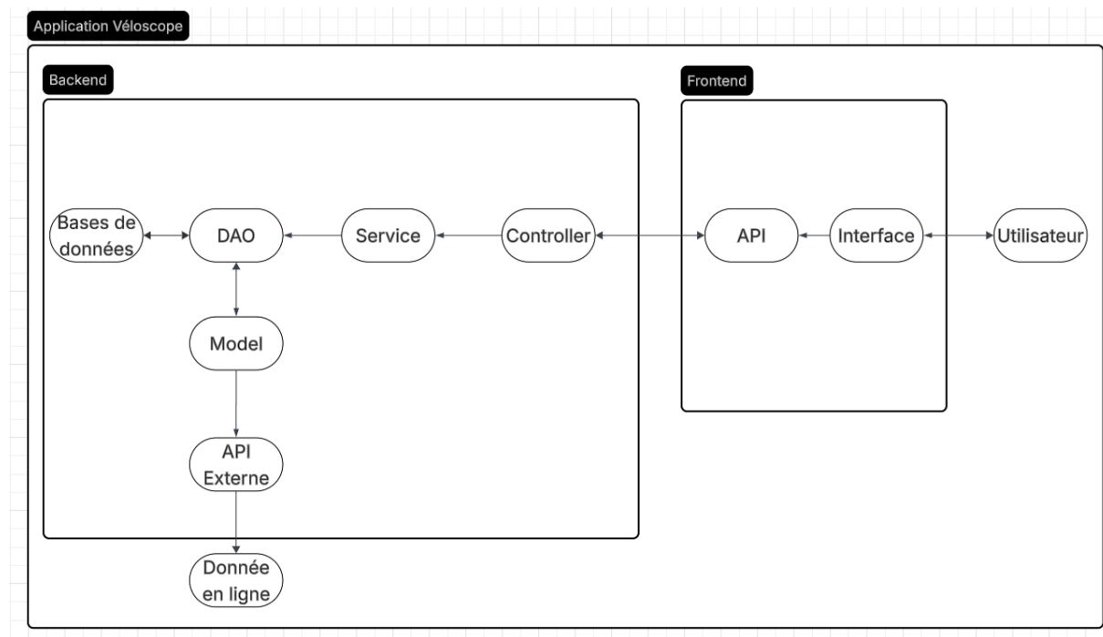
FIGURE 2 : Diagramme d'architecture
