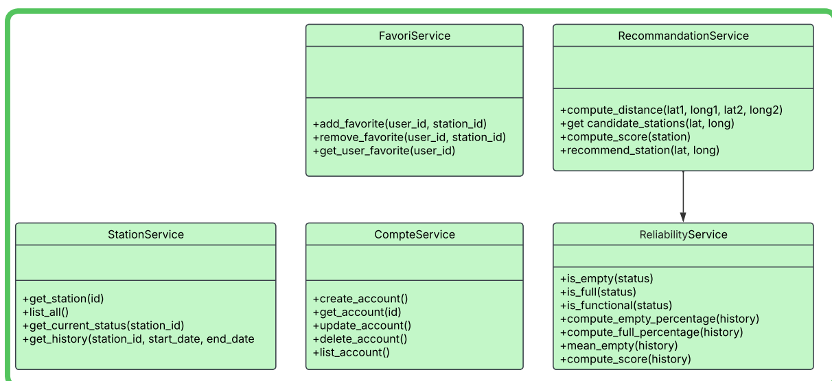
FIGURE 8 : Diagramme de classes du module Service
