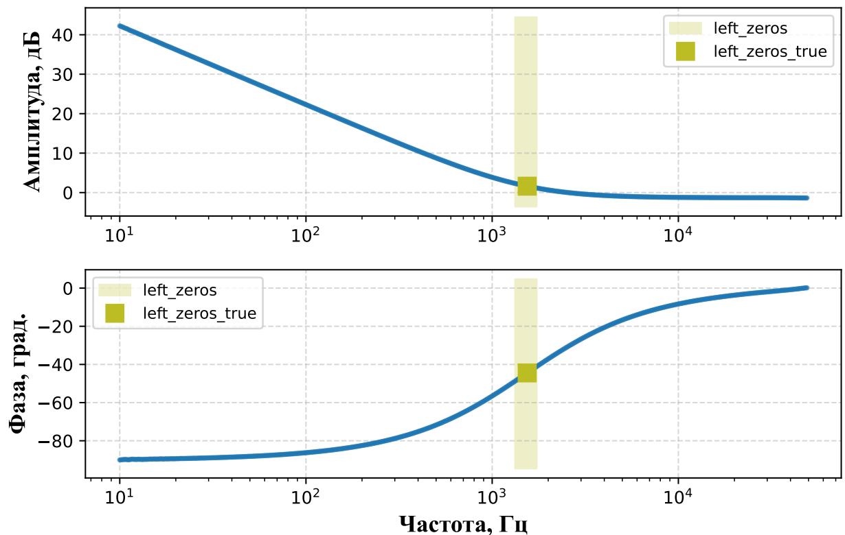
Рисунок 3.5. Частотные характеристики ПИ-регулятора контура регулирования тока (внутрисхемное измерение)
