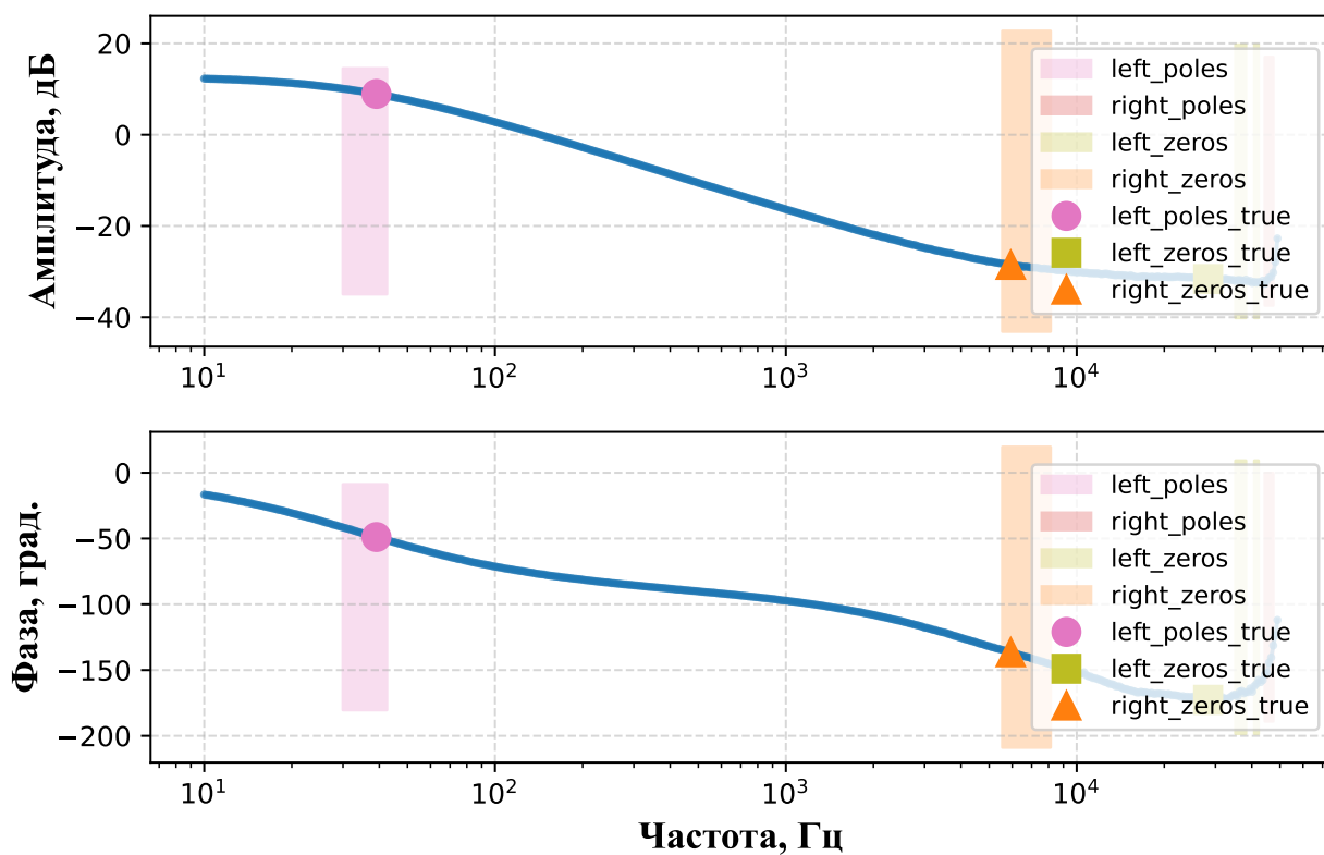
Рисунок 3.9. Частотные характеристики коэффициента преобразования тока в напряжение при введенной задержки времени (внутрисхемное измерение)
