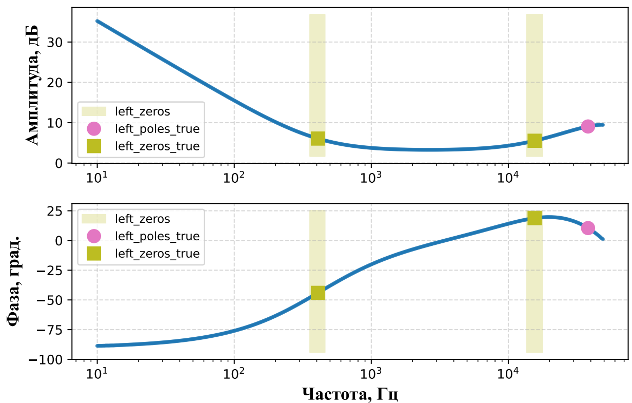
Рисунок 3.7. Частотные характеристики ПИД-регулятора контура регулирования тока (внутрисхемное измерение)
