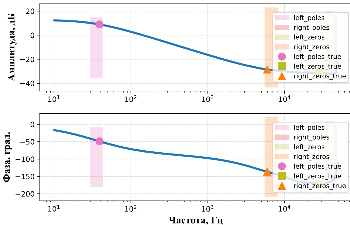
Рисунок 3.8. Частотные характеристики коэффициента преобразования тока в напряжение (внутрисхемное измерение)
