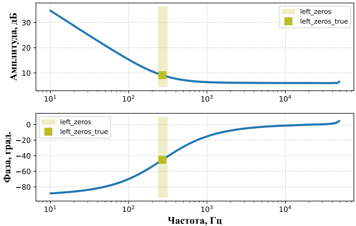
Рисунок 3.6. Частотные характеристики ПИ-регулятора контура стабилизации напряжения (внутрисхемное измерение)
