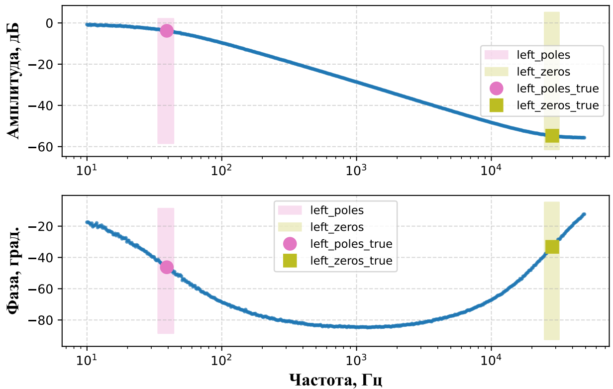
Рисунок 3.11. Частотные характеристики выходного импеданса источника питания в режиме стабилизации тока (измерение внешним анализатором)
