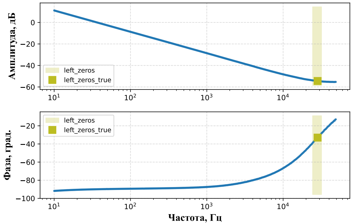
Рисунок 3.10. Частотные характеристики выходного импеданса выключенного источника питания (измерение внешним анализатором)
