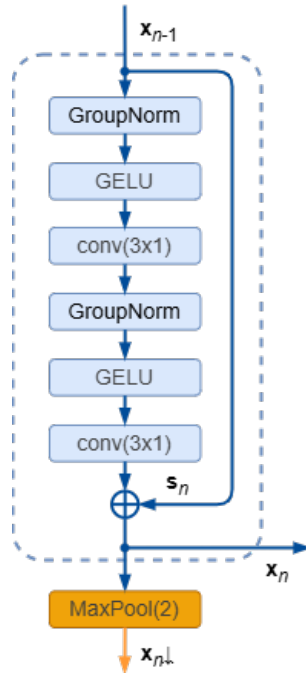
Рисунок 3.3. Блок-схема bottleneck-алгоритма
